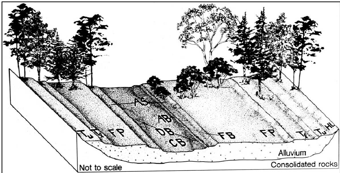
Obr. 5: Digram znázorňující lužní plochy na dně údolí: CB – dno říčního koryta, DB – šterková lavice v korytě toku, AS – horní okraj koryta (horní povodňové koryto), AB – břeh, agradační val, FP – údolní niva, TL – nižší terasa, TU – vyšší terasa, HL – údolní svah (Hupp, C. R., Osterkamp, W. R., 1985)
