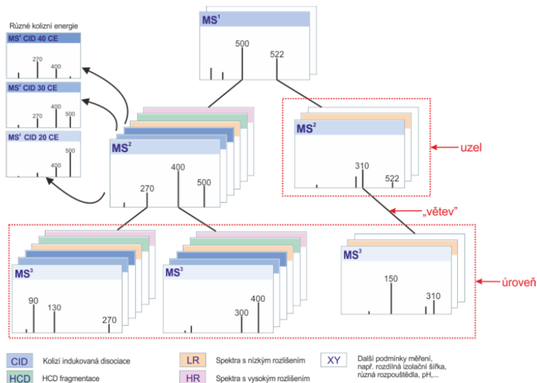
Obrázek 2. Schéma spektrálního stromu. Větvě spojují prekurzorové ionty s uzly dceřiných spekter, měřených při různých podmínkách fragmentace. Zobrazena je fragmentace do úrovně MS 3 (upraveno podle www.mzcloud.org , HighChem, SK).
