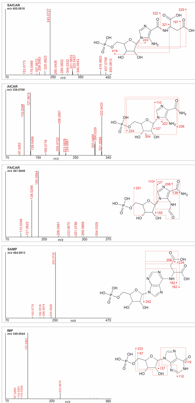
Obrázek 10. MS 2 fragmentační spektra ribotidů SAICAR, AICAR, FAICAR, SAMP a IMP. Struktura fragmentované molekuly je znázorněna vedle každého hmotnostního spektra a je v ní zobrazeno nejvýše 6 fragmentů s nejvyšší intenzitou.
