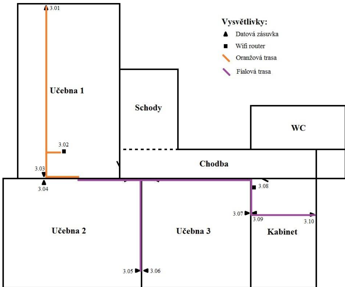
Obrázek 14 Trasy kabeláže 3NP (vlastní tvorba)
