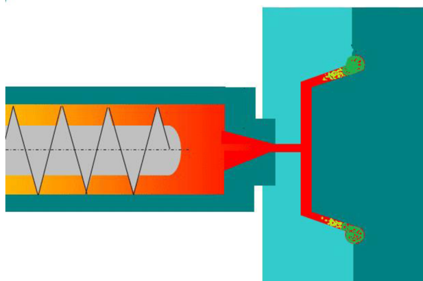
Obr. 31: Schéma ochlazování [32].
