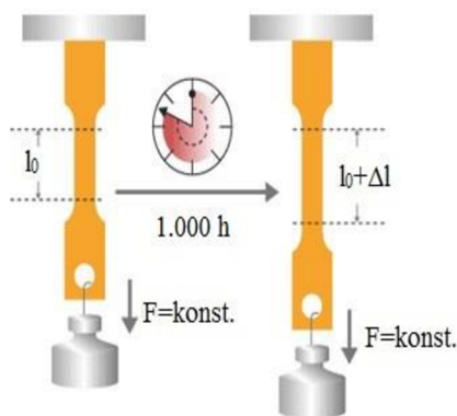
Obr. 13: Princip křípkové chování v tahu [2].
