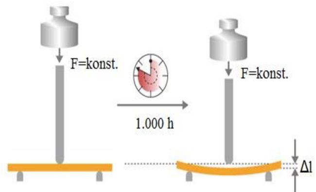
Obr. 14: Princip křípového chování v ohybu při třibodovém zatížení [1].
