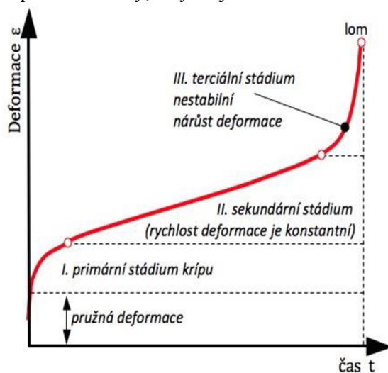
Obr. 12: Obecná křípková křivka [2].
