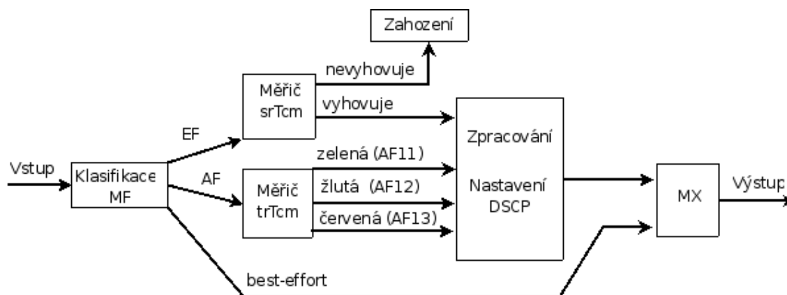
Obr. 4.1: Zpracování paketů ve vstupním směru
