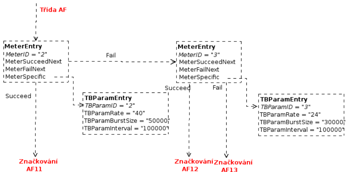
Obr. 4.4: Struktura měřiče trTCM
