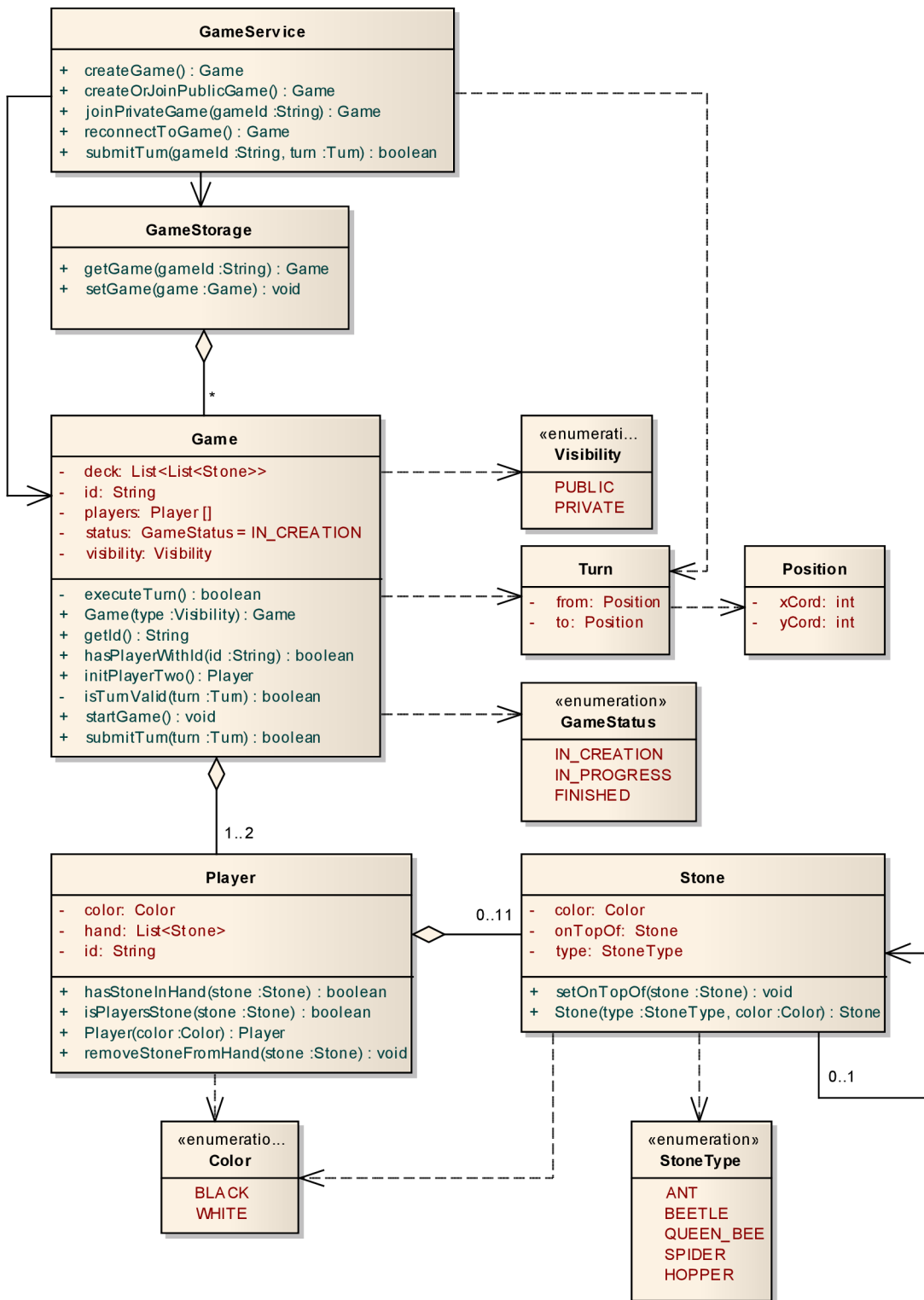
Obrázek 17: Diagram tříd
