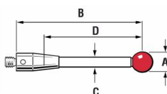
Obr. 10 Rozměry doteku [6]
