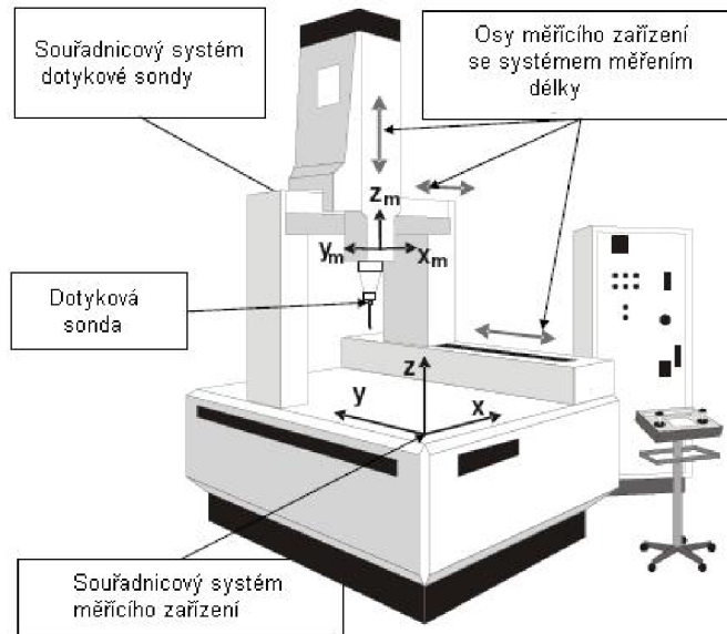
Obr. 7 Detail konstrukce [2]
