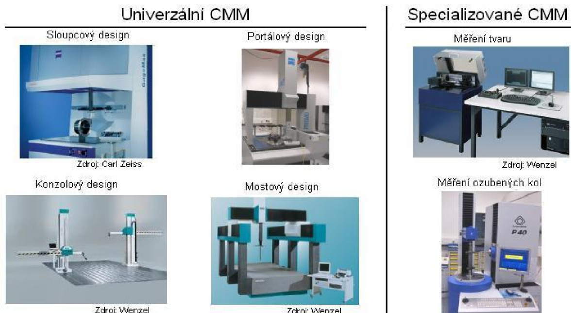
Obr. 4 Typy konstrukcí [2]
