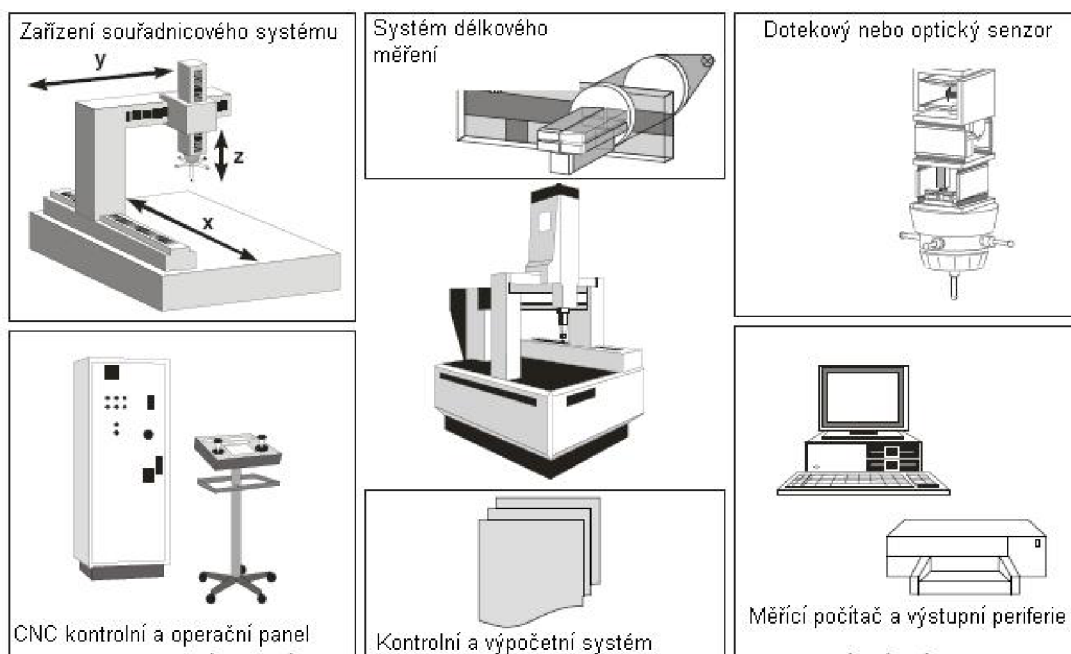
Obr. 3 Měřicí řetězec [2]
