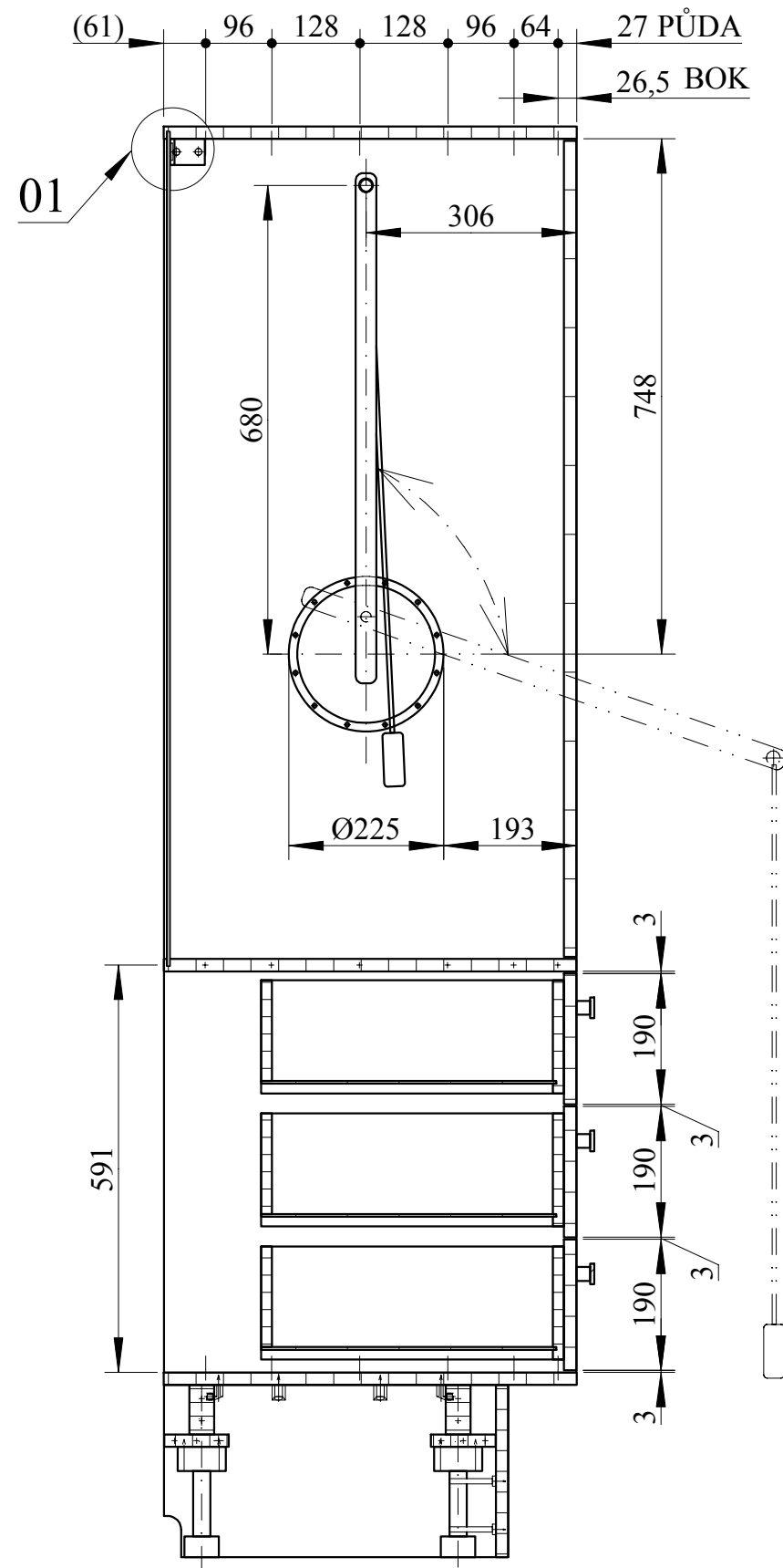
A-A (1:10)
