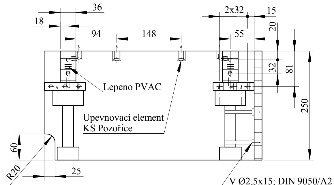
Sokl (1:5)
