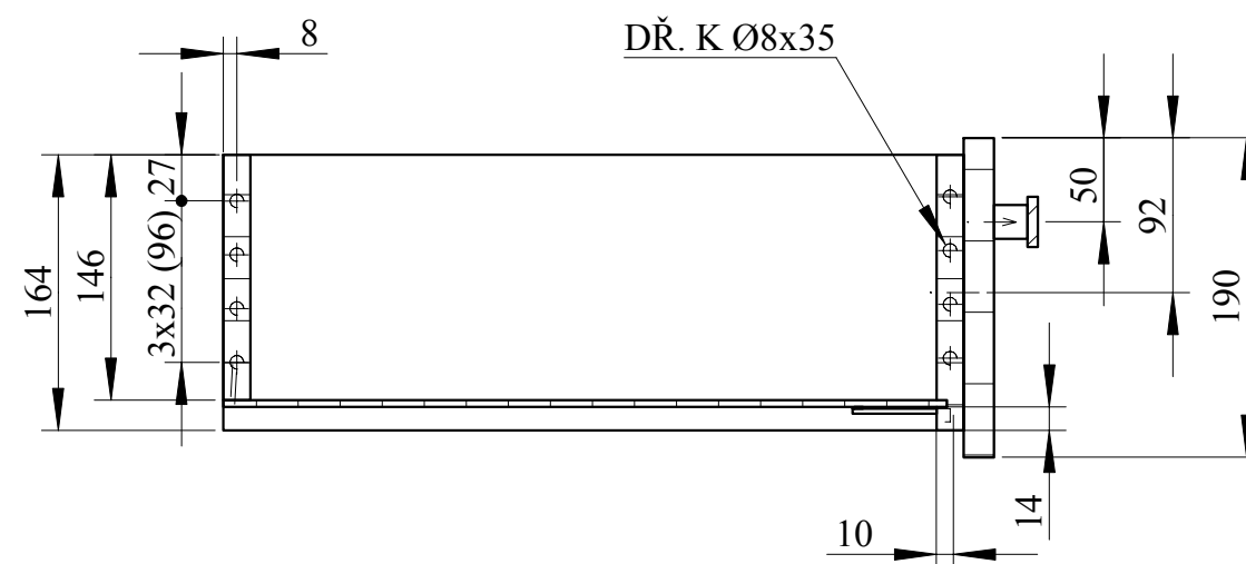
Zásuvka (1:5)
