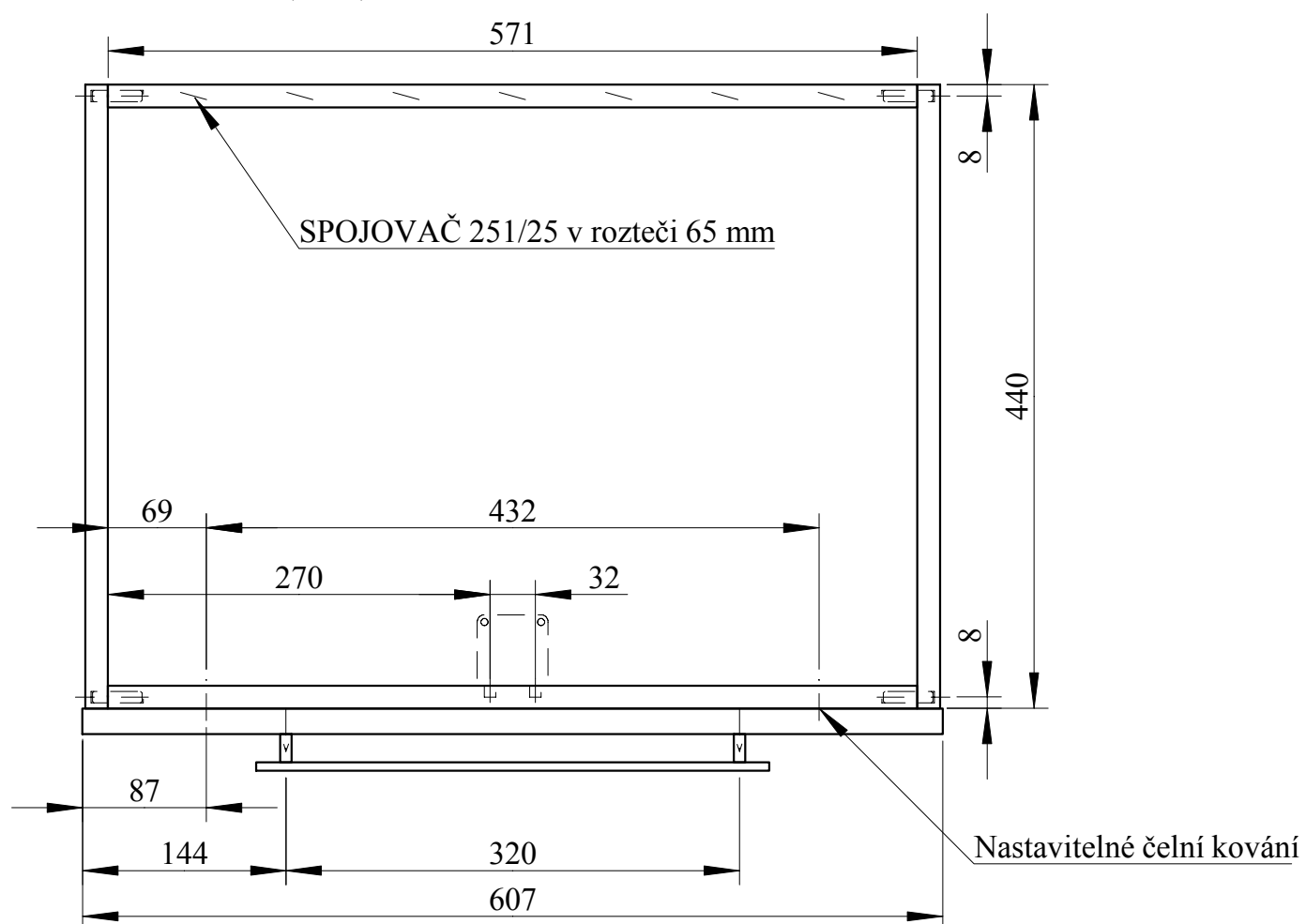
Zásuvka (1:5)
