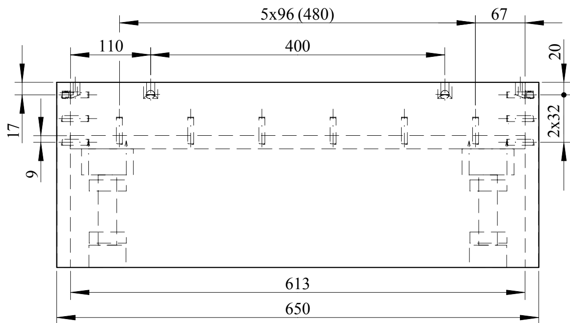
Sokl (1:5)
