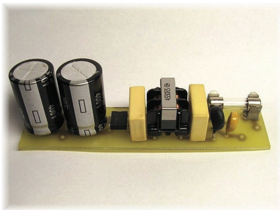
Obr. 4.9: Filtr
