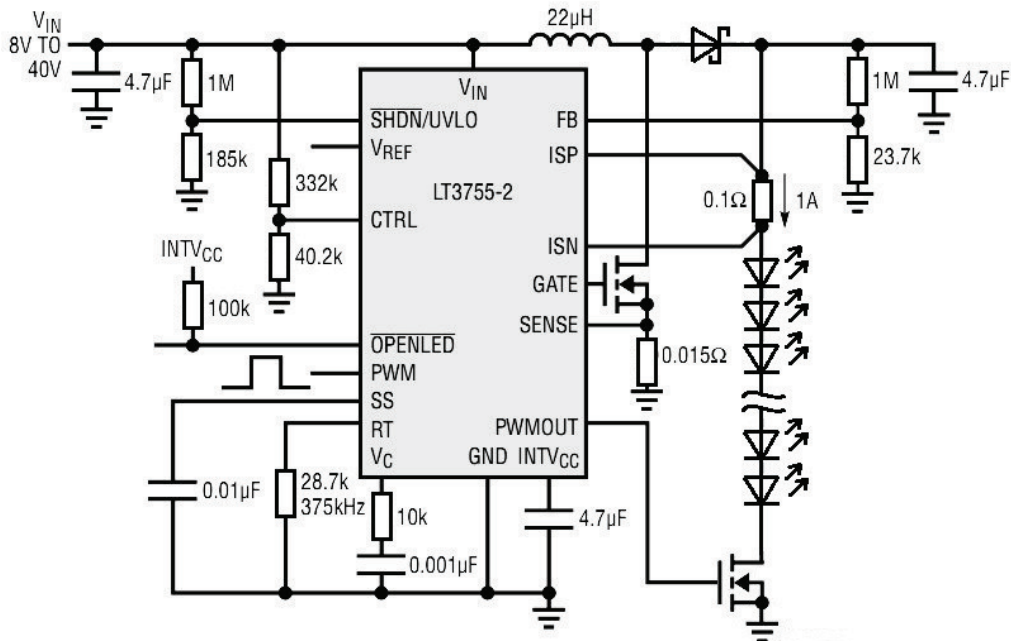
Obr. 3.1: Napájecí obvod pro napájení 50W LED světlometu s LT3755 [21]
