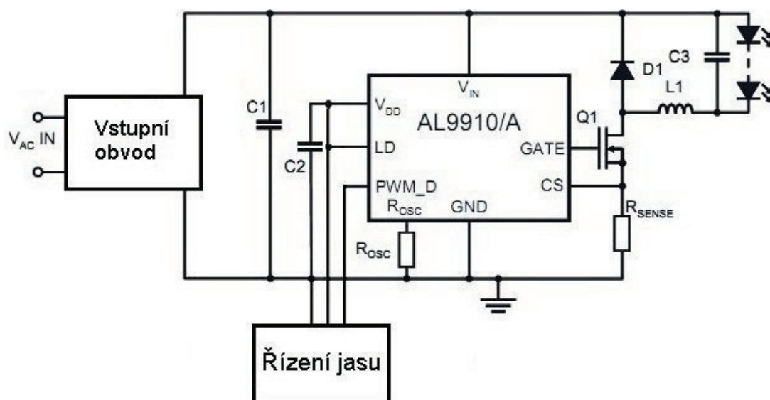
Obr. 4.1: Schéma obvodu s AL9910
