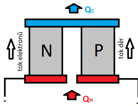
Obr. 1.10: Peltierův článek
