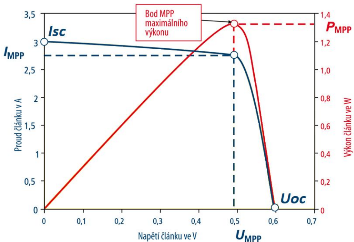
Obr. 1.6: Zatěžovací a výkonová charakteristika FV článku
