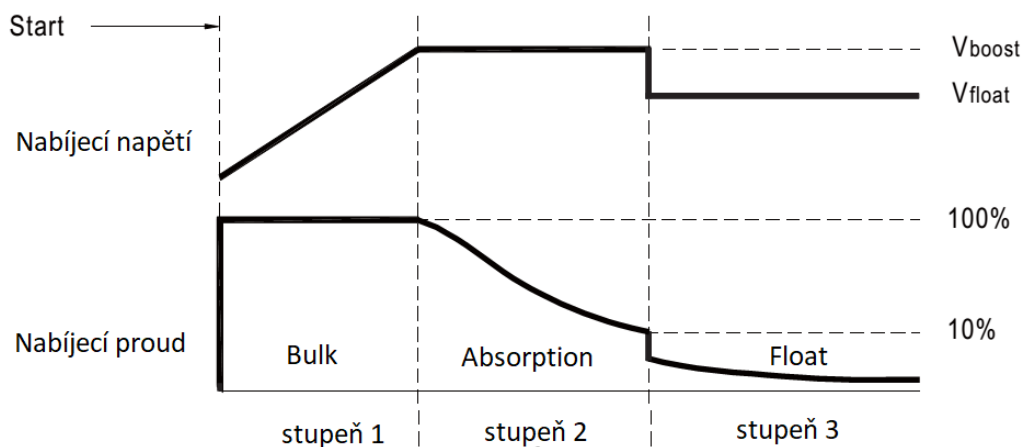
Obr. 4.1: Třístupňové nabíjení [45]
