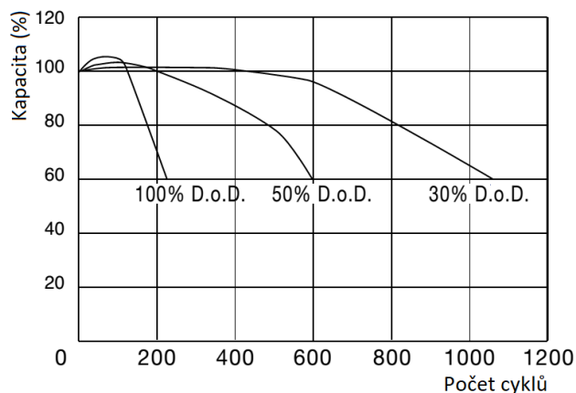
Obr. 4.5: Závislost kapacity AKU na počtu cyklů [34]
