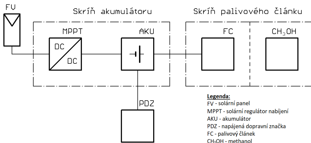
Obr. 3.2: Blokové schéma sestavy
