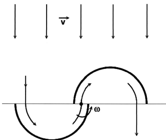
Obr. 1.20: Savoniův motor [1]
