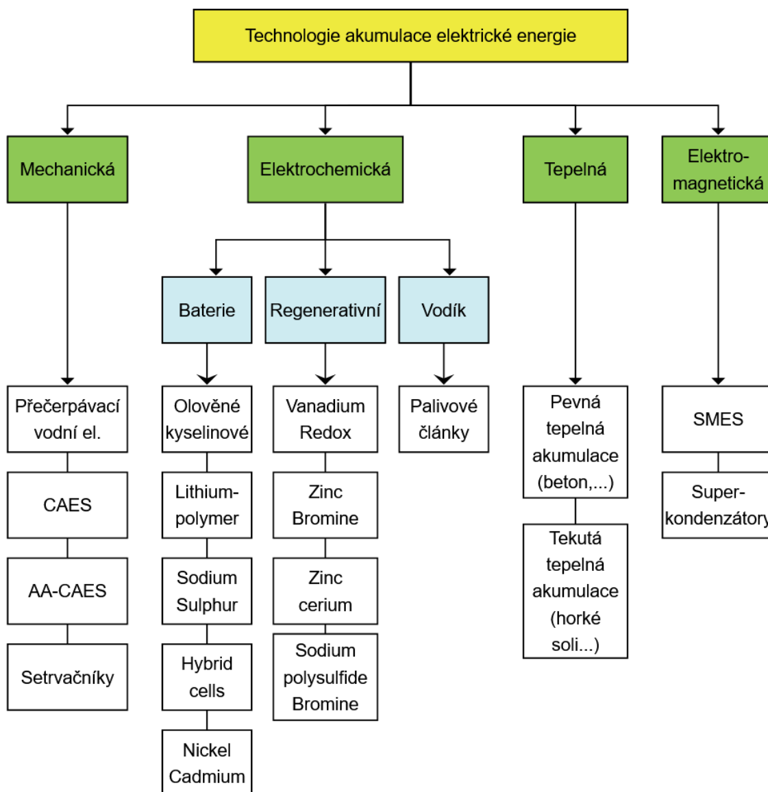
Obr. 2.1: Rozdělení akumuláčních soustav [1]
