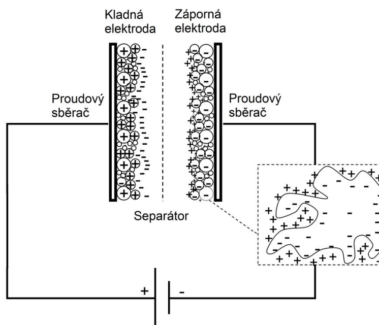
Obr. 2.4: Struktura superkondenzátoru [32]
