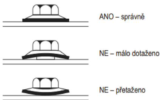
Obr. 8.6 schéma správného dotažení šroubů
