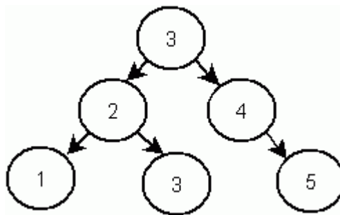
Obr. 18: Náhodně vygenerovaný binární vyhledávací strom
