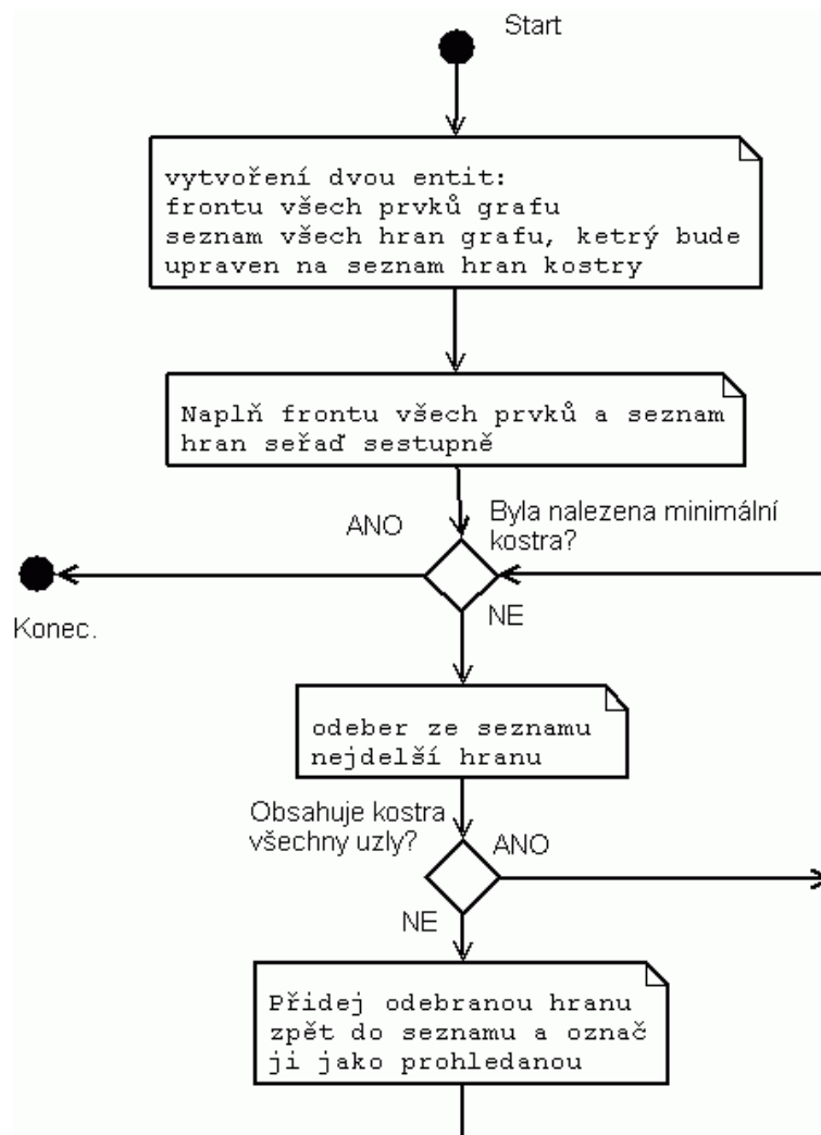
Obr. 28: Vývojový diagram Kruskalova hladového algoritmus. Varianta s odebíráním hran.
