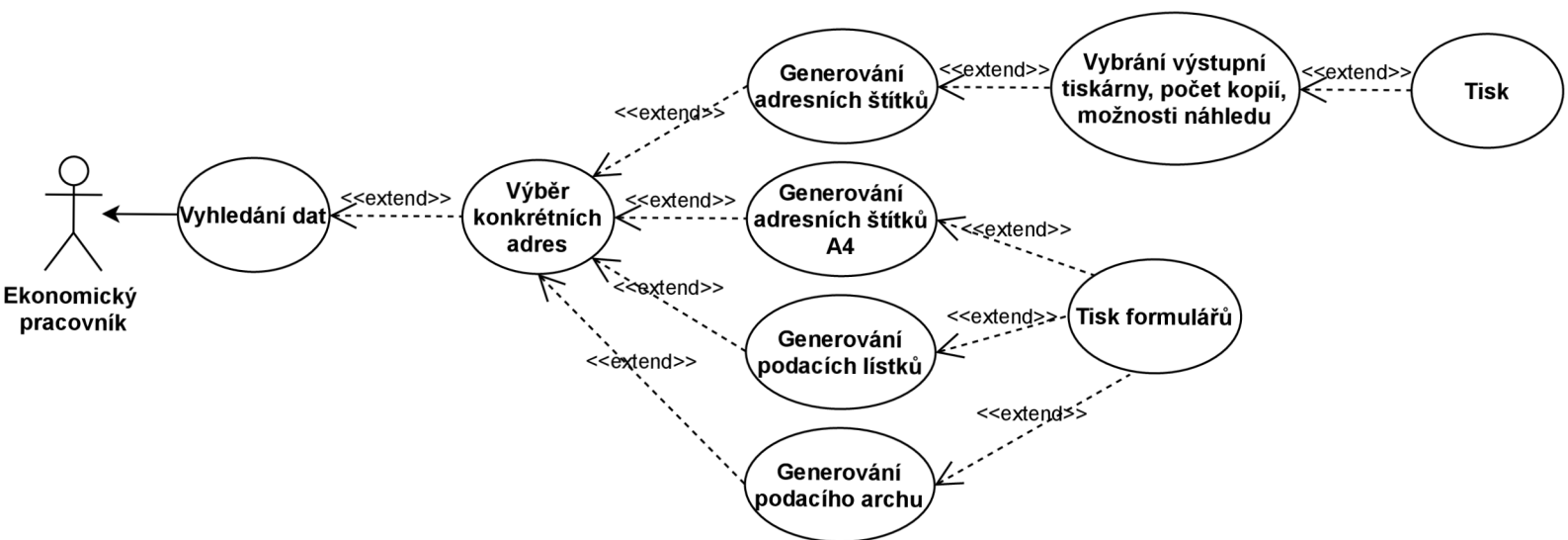
Obrázek 4.6: Diagram případu užití aplikace.
