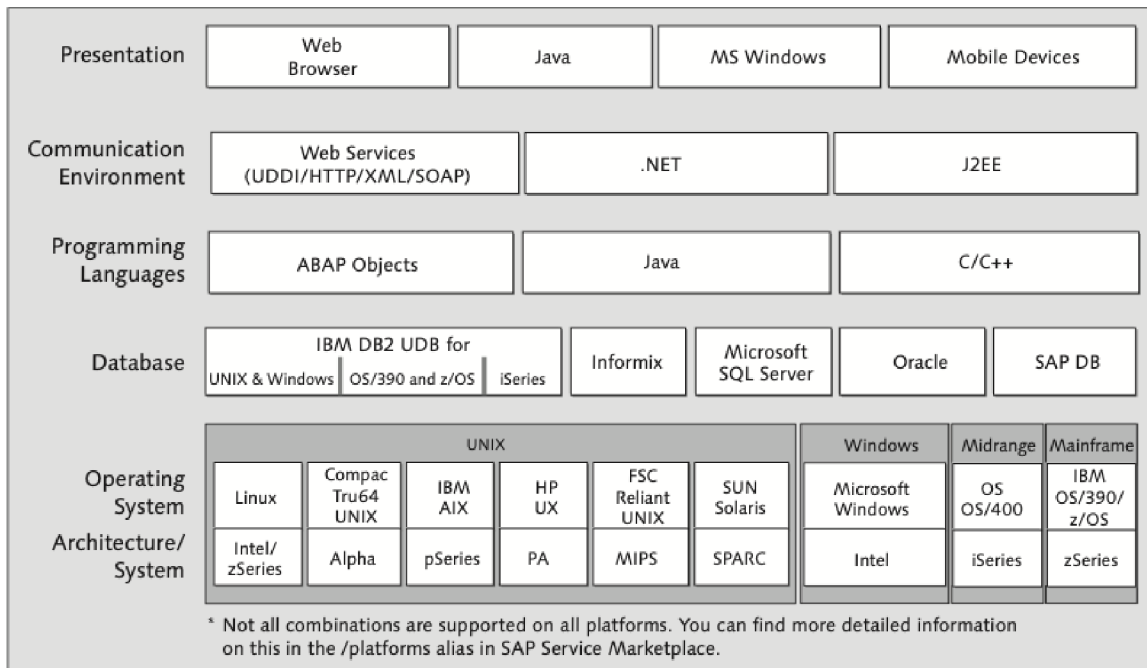
Obrázek 2.3: Přehled technologií podporující SAP[9].
