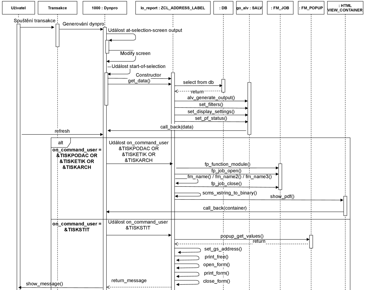
Obrázek 4.8: Sekvenční diagram řízení tisku formulářů.
