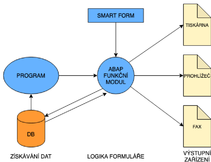
Obrázek 3.3: Architektura SAP Smart Form.
