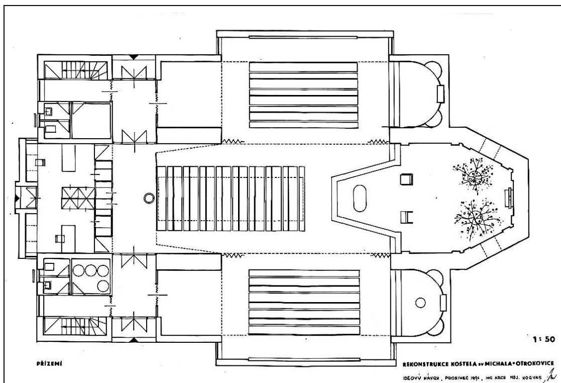
Obr. 81: Mojmir Korvas – Ideový návrh rekonstrukce kostela sv. Michaela (1991)
