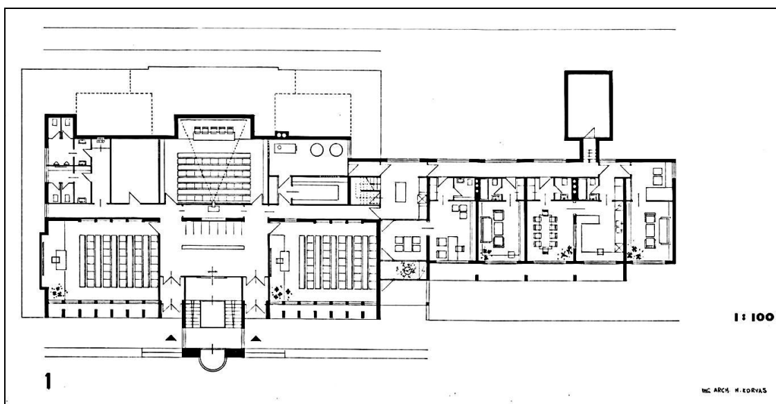
Obr.62: Mojmir Korvas – Ideový návrh kostela v Otrokovcích, suterén (1970)
