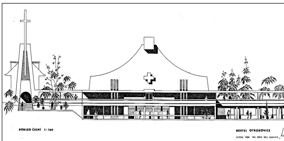
Obr. 82: Mojmir Korvas – Studie kostela sv. Vojtěcha v Otrokovicích, varianta kostela bez věže (1992)
