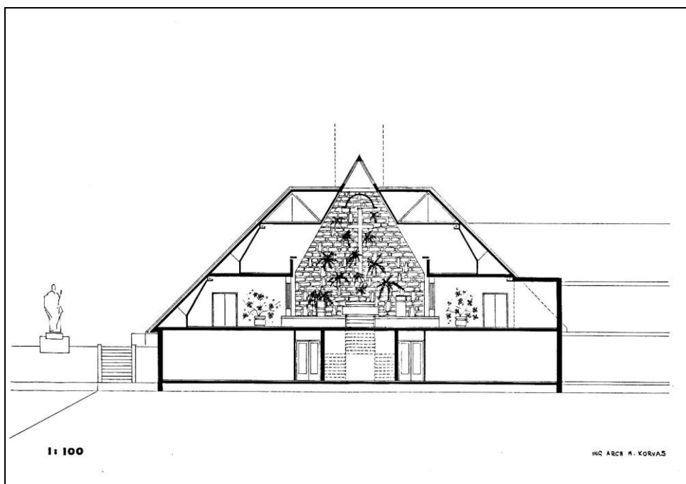
Obr. 63: M. Korvas – Ideový návrh kostela v Otrokovicích, pohledový řez k oltáři (1970)
