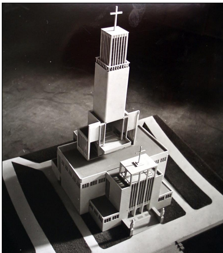
Obr. 12: Vladimír Karfík – Maketa návrhu kostela v Otrokovcích (1936)
