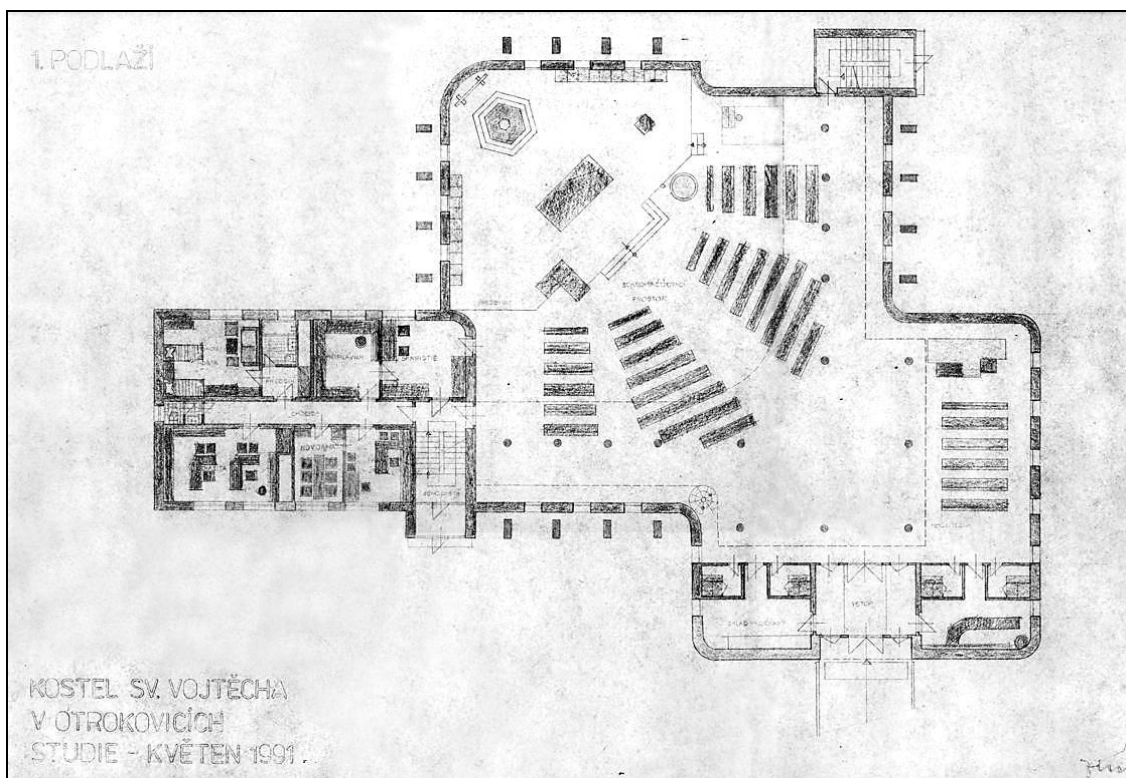
Obr. 78: Josef Tat'ák – Studie kostela sv. Vojtěcha, I. podlaží (1991)
