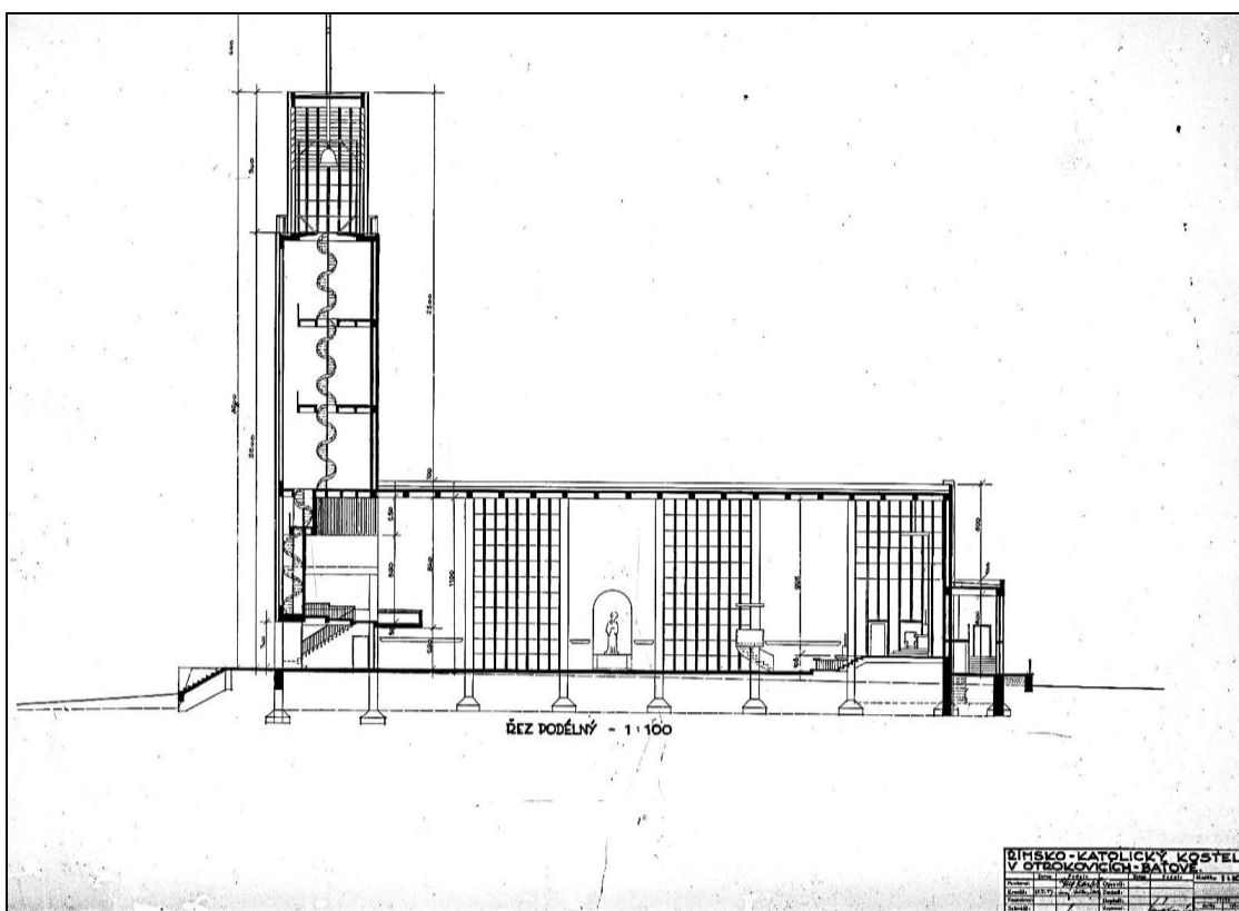
Obr. 20: V. Karfik – Návrh kostel v Otrokovcích-Baťově U boží muky, podélný řez
