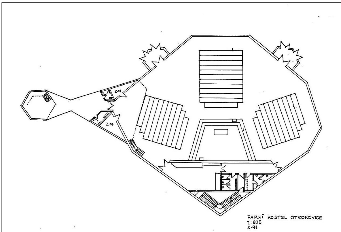
Obr. 80: Tomáš Černoušek – Návrh na farní kostel sv. Vojtěcha v Otrokovicích (1991)
