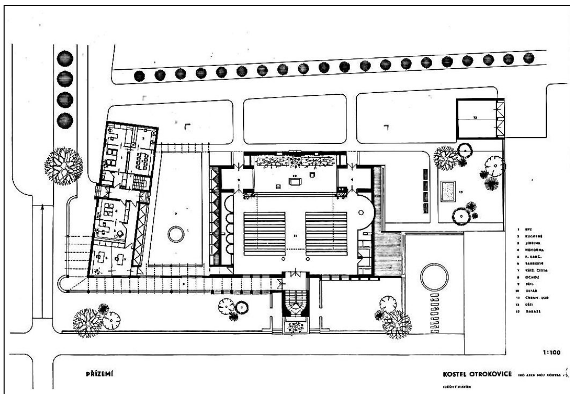
Obr. 68: M. Korvas - Ideový návrh kostela v Otrokovicích, 3. verze, přízemí (1970)
