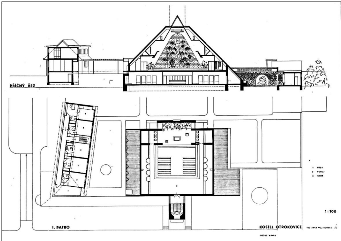
Obr. 69: M. Korvas - Ideový návrh kostela v Otrokovicích, 3. verze, 1. patro (1970)
