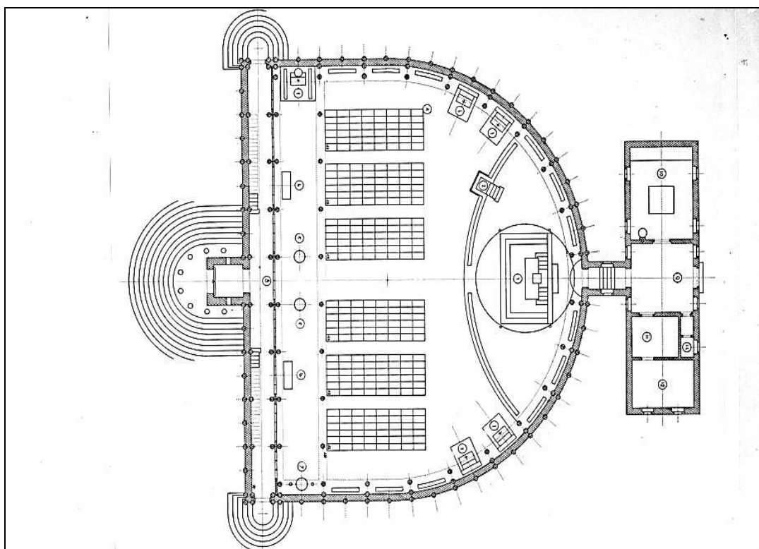
Obr. 47: O. Rothmayer - Soutěžní návrh kostela a památníku, půdorys (1940)
