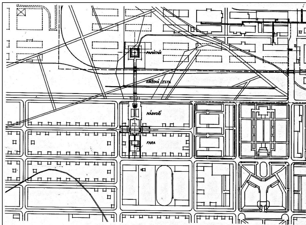
Obr. 28: Umístění soutěžních návrhů kostela a památníku T. Bati v Baťově - výřez situace Vladimír Karfik (1940)
