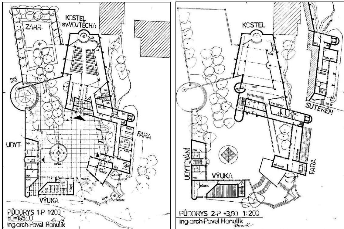
Obr. 73: Pavel Hanulík – Soutěžní návrh na kostel sv. Vojtěcha v Otrokovicích, půdorysy 1. a 2. patro (1990)
