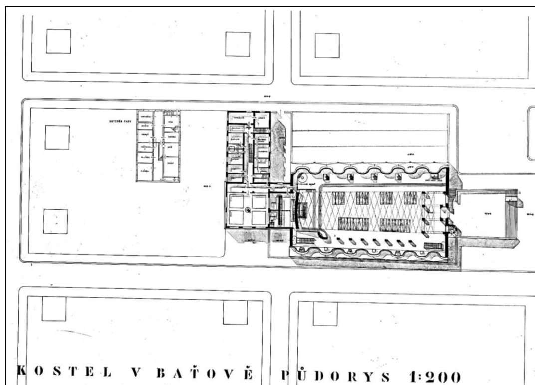
Obr. 30: J. Sokol – Vítězný soutěžní návrh kostela a památníku T. Bati v Bařově, půdorys (1940)
