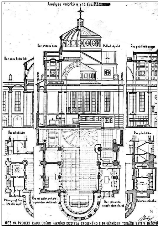
Obr. 37: Karel Engel – Soutěžní návrh kostela a památníku T. Bati v Bařově (1940)
