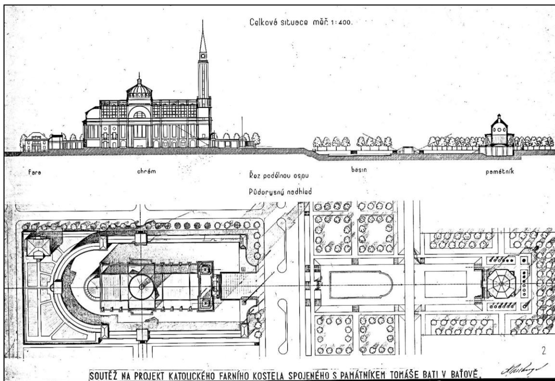
Obr. 35: K. Engel – 3. místo, soutěžní návrh kostela a památníku T. Bati v Baťově (1940)
