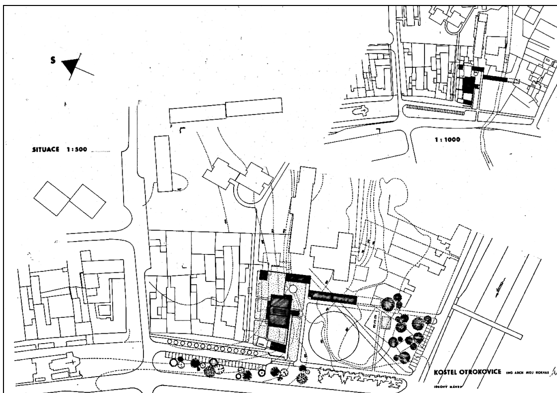
Obr. 66: M. Korvas - Ideový návrh kostela v Otrokovicích, 3. verze, situace (1970)
