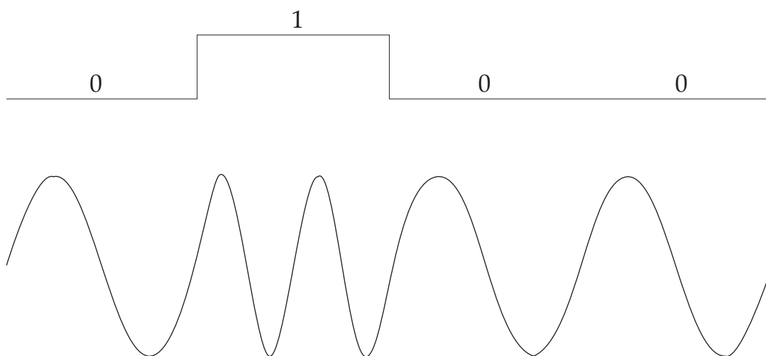
Obr. 1.3: Modulace FSK.
