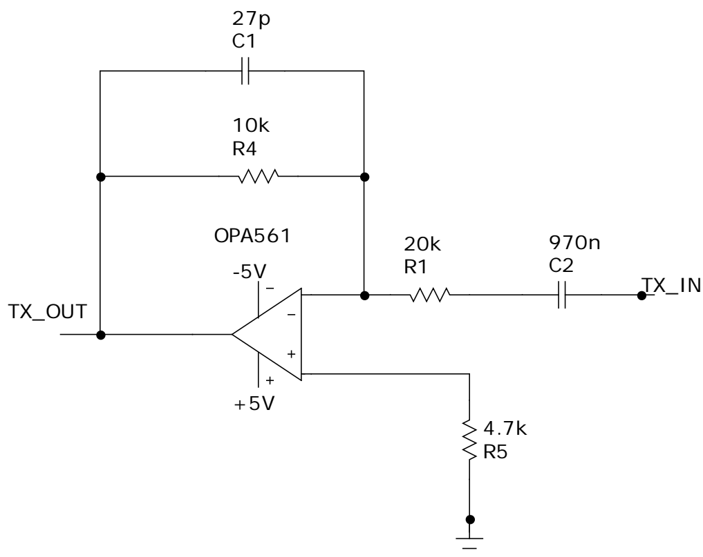
Obr. 2.7: Schéma zapojení filtru pro přijímač.
