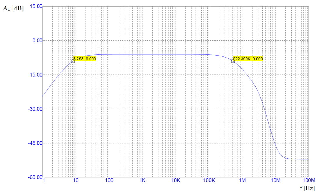
Obr. 2.8: Graf aktivního filtru pro vysílač.
