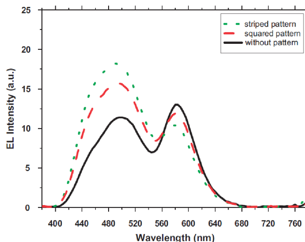
Obr. 8: Porovnanie konvenčného a štrukturovaných panelov [2]
