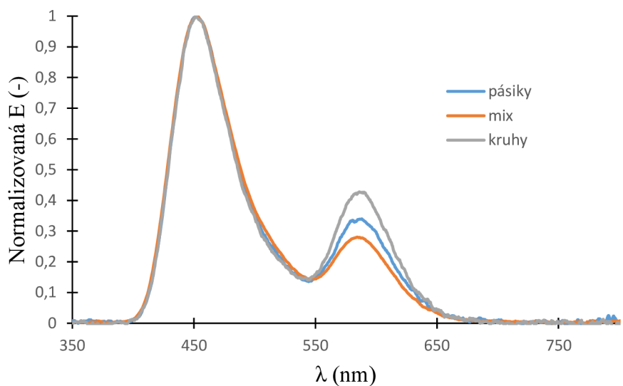
Obr. 20: Porovnanie normalizovaných dát zmesi, pásikov a kruhov (250 V, 10 000 Hz)
