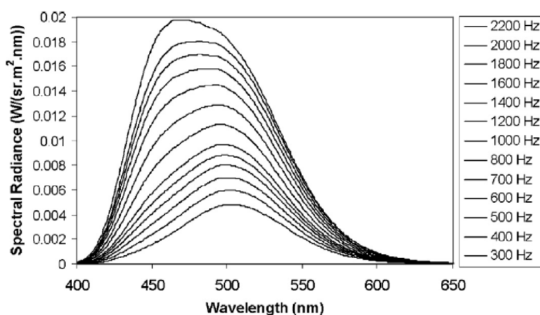
Obr. 5: Vplyv frekvencie na farbu emisie [18]
