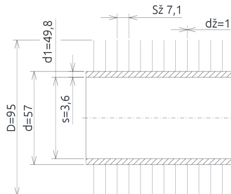
Obr. 5-7 Trubky VT_VYP
