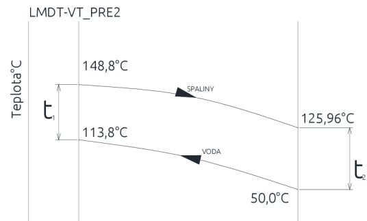
Obr. 5-32 LMDT VT EKO11
