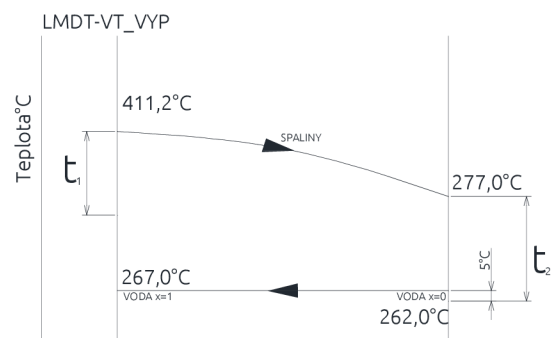
Obr. 5-8 LMDT VT_VYP
