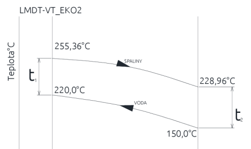
Obr. 5-15 LMDT VT EKO2
