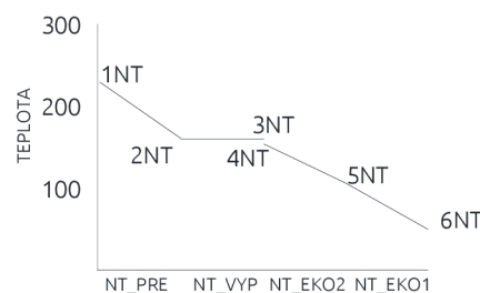
Obr. 4-5 Průběh teplot NT části
