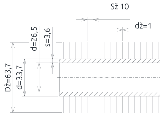
Obr. 5-31 Trubky VTEKO11
