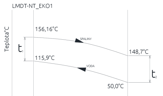
Obr. 5-29 LMDT NT EKO 2
