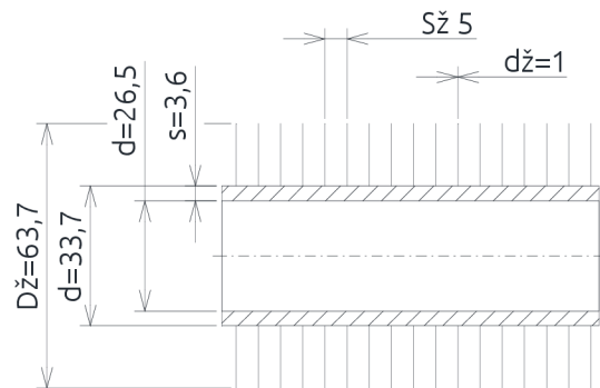
Obr. 5-28 Trubky NT EKO 2
