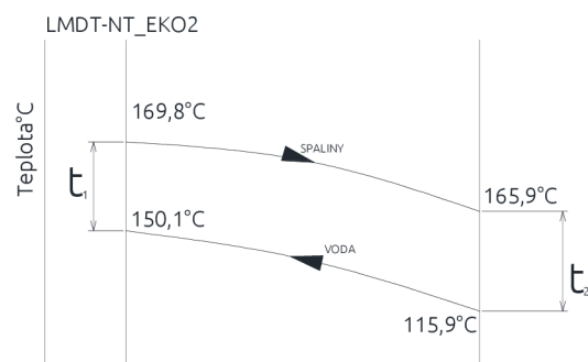
Obr. 5-23 LMDT NT_EKO2
