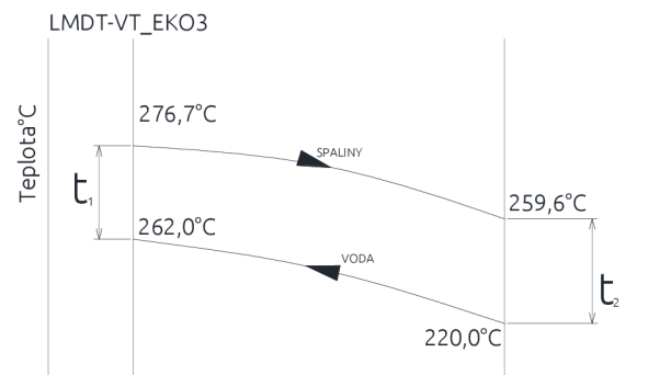
Obr. 5-10 LMDT VT_EKO3
