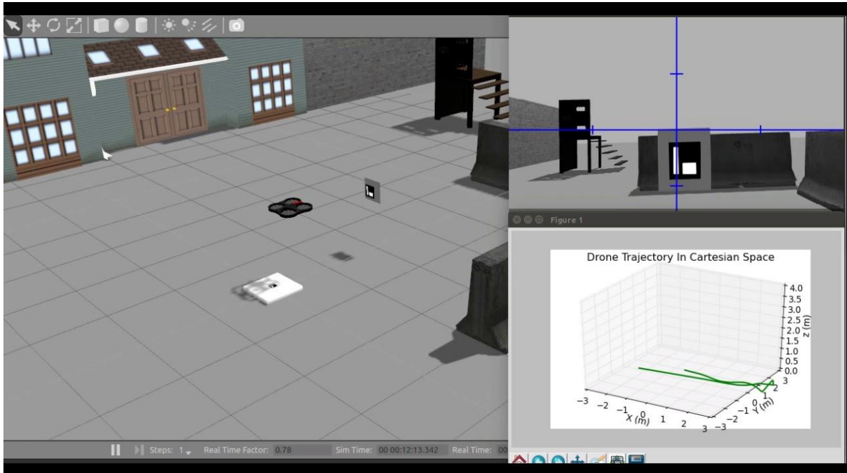
Obrázek 6 Simulace dronu v prostředí Gazebo [21]
