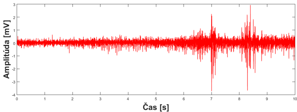
Obrázok 12. 21 : EMG biosignál, koniec nočnej jazdy, 10s.
