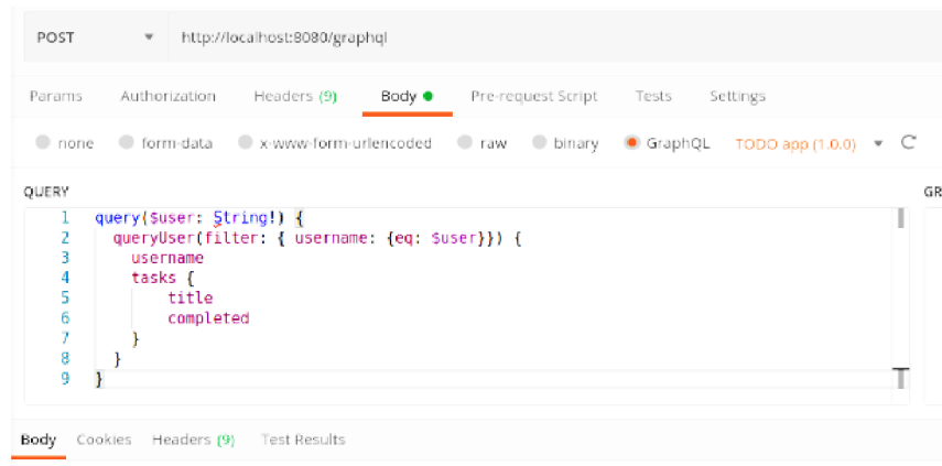
Obr. 3. Volání GraphQL endpointu v Postmanu.
