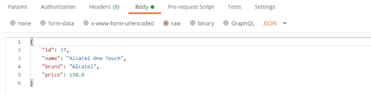
Obr. 12. Tělo požadavku.
