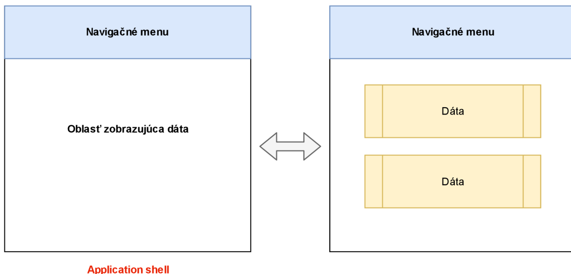
Obrázok 1: Application shell
