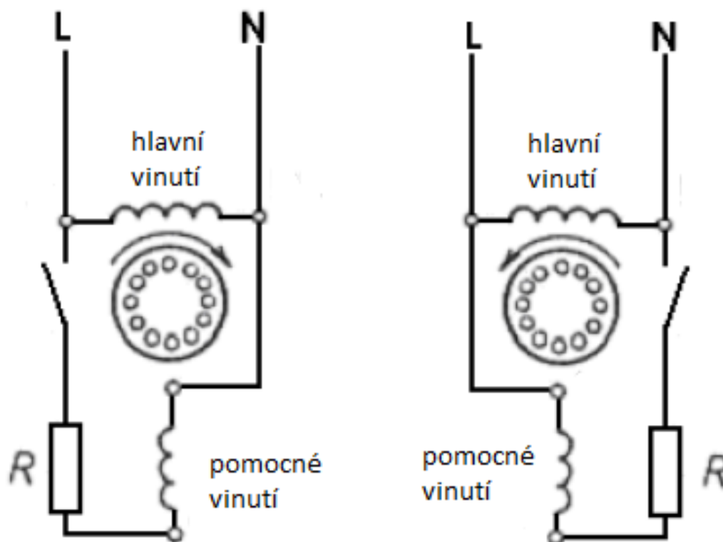
Obrázek 13 Zapojení jednofázového asynchronního motoru s odporovým rozběhem
