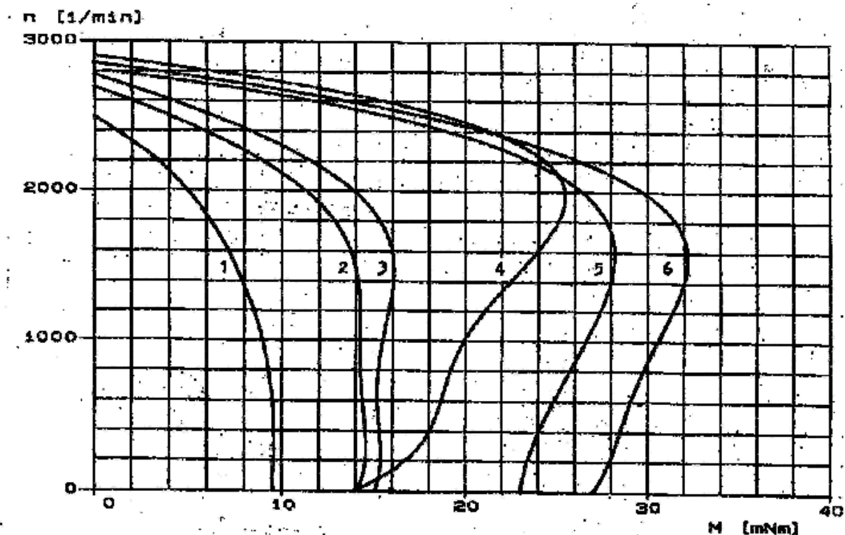
Obrázek 11 Momentová charakteristika A24NF325L motorku [3]
