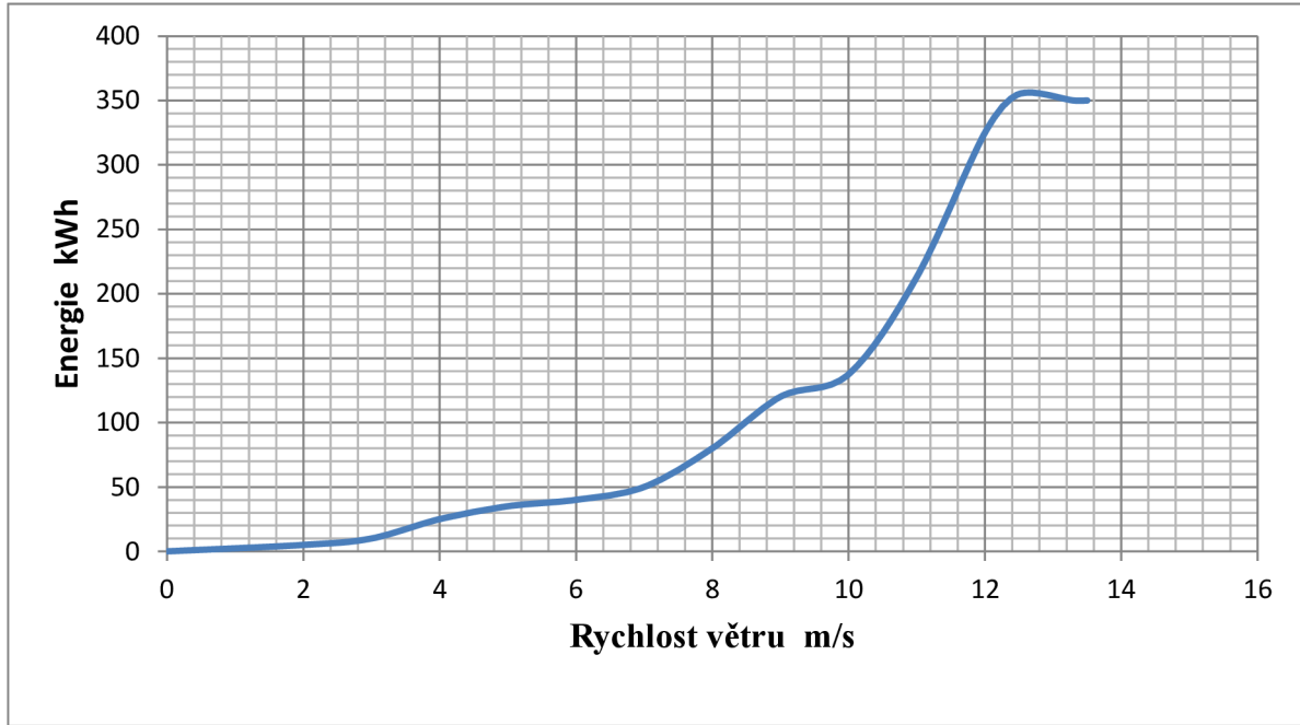
Obr. 5-2 Výkonová charakteristika větrné elektrárny VTE200.H1, modifikováno z [15]
