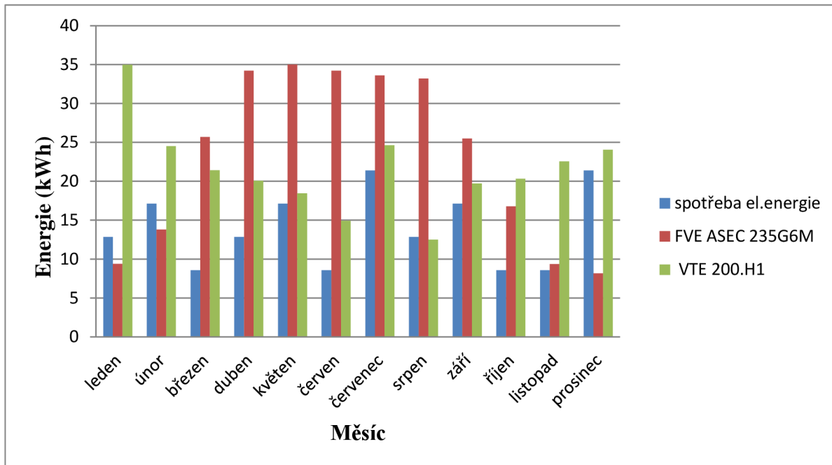
Obr. 5-3 Přírůstek energie FVE a VTE v porovnání se spotřebou elektrické energie
