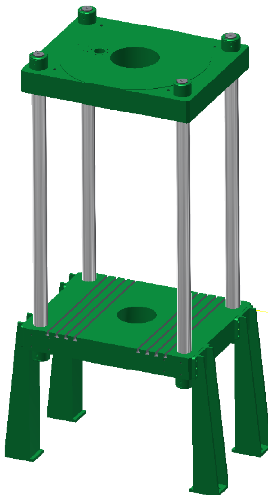
Obr. 1.4 Rám lisu.
