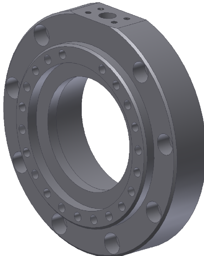
Obr. 2.1 Příruba.
