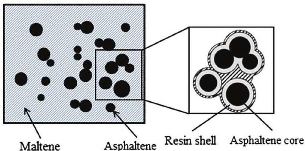
Obrázek 1: Schéma koloidní struktury asfaltového pojiva [35]
