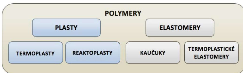
Obrázek 9: Rozdělení polymerů [14]
