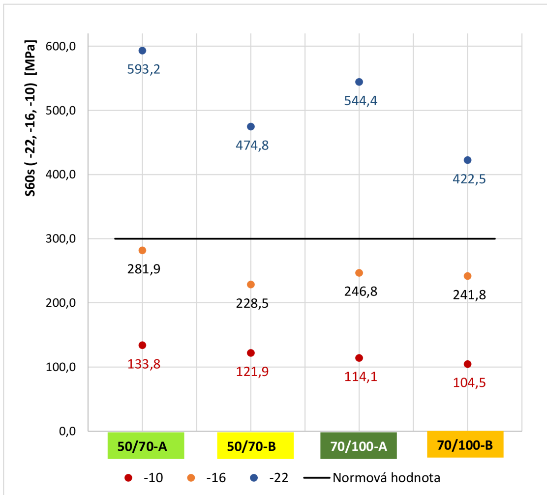
Graf 27: Modul tuhosti silničních asfaltů po RTFOT+PAV
