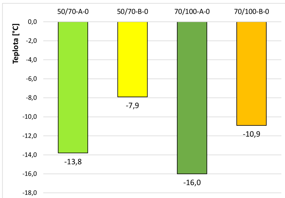
Graf 32: Kritické teploty ze m60s silniční asfaltu po RTFOT+PAV
