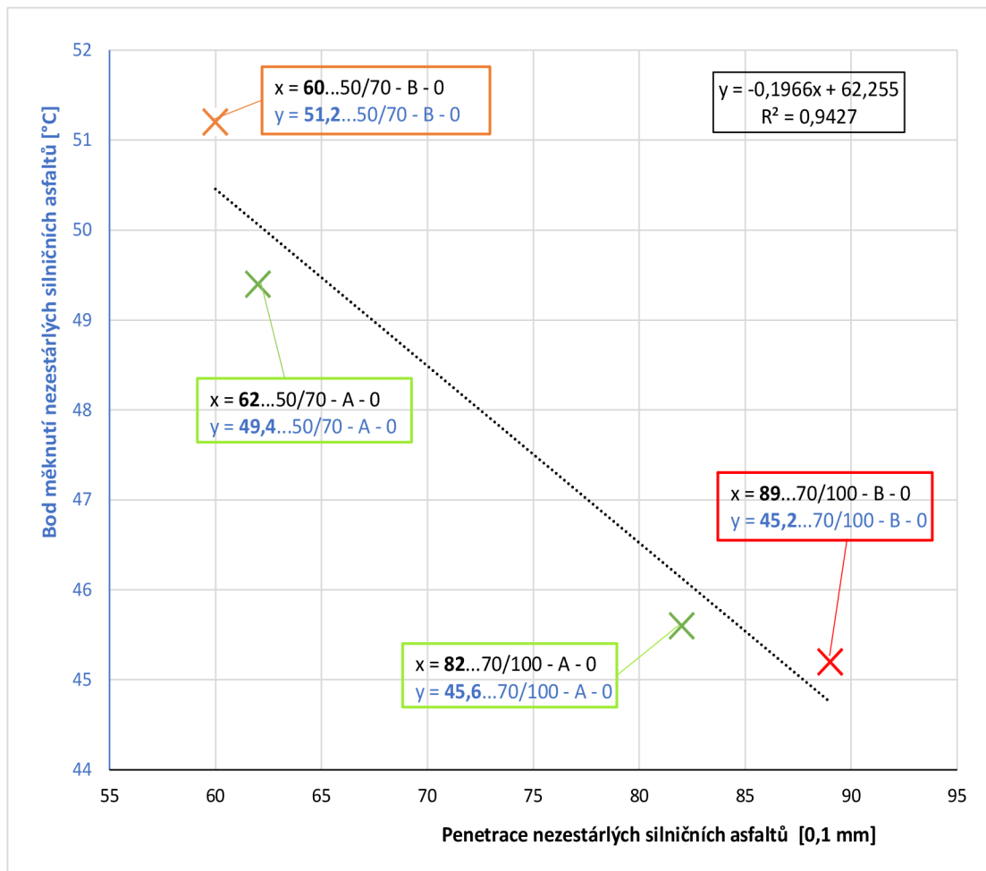
Graf 38: Závislost mezi penetrací a bodem měknutí nezestárlého silničního asfaltu
