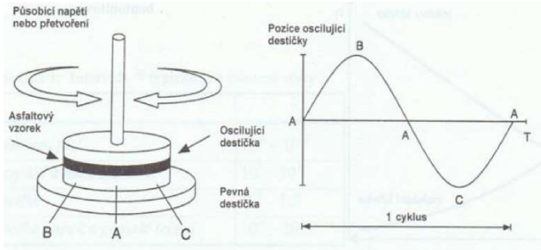
Obrázek 24: Princip DSR [36]
