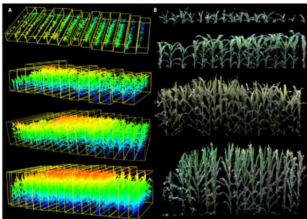
Obr. 8 Struktura porostu vytvořená pomocí skenování Lidarem
