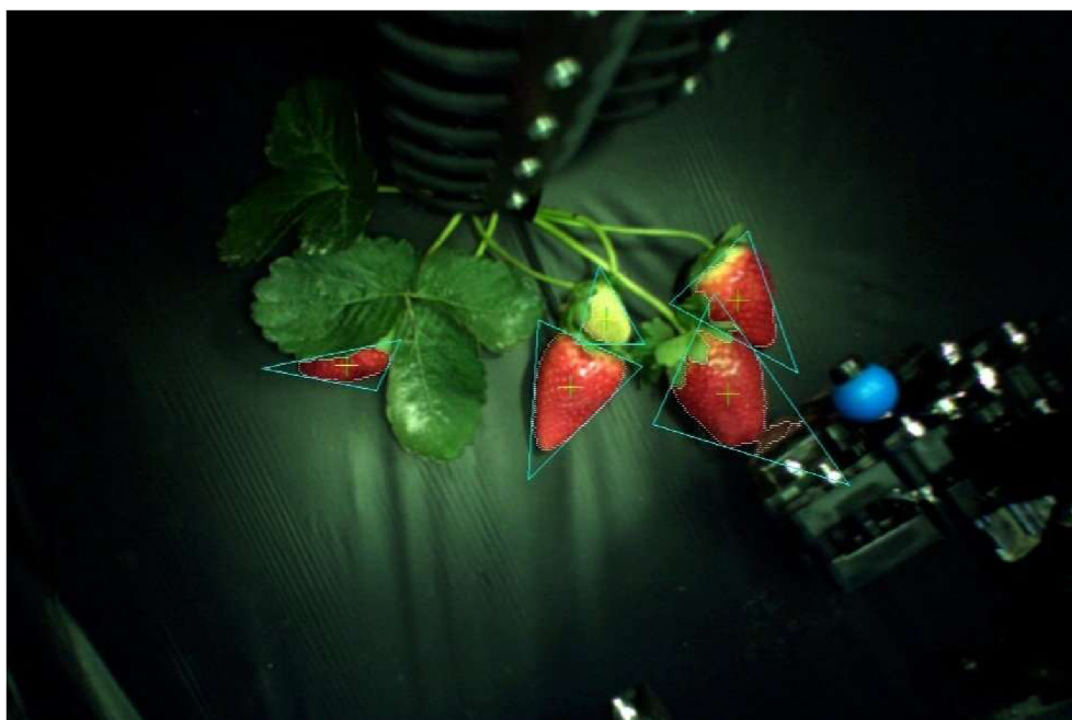
Obr. 23 Optická identifikace plodů a zhodnocení stavu zralosti dle AI
