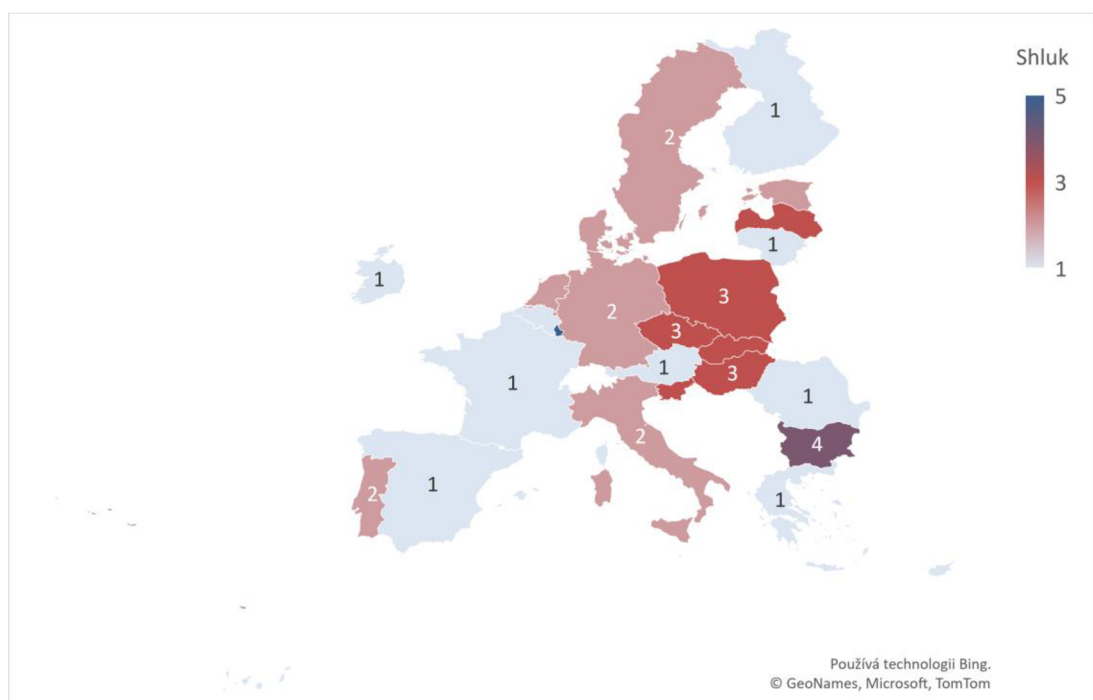
Obrázek 2: Mapa shluků (1)
