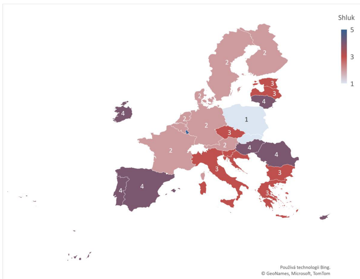
Obrázek 4: Mapa shluků (1)
