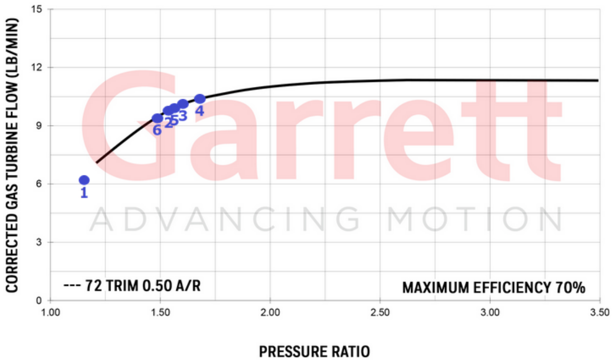
Obr. 51 Pracovní body zakreslené v charakteristice vysokotlaké turbíny [4] - upraveno
