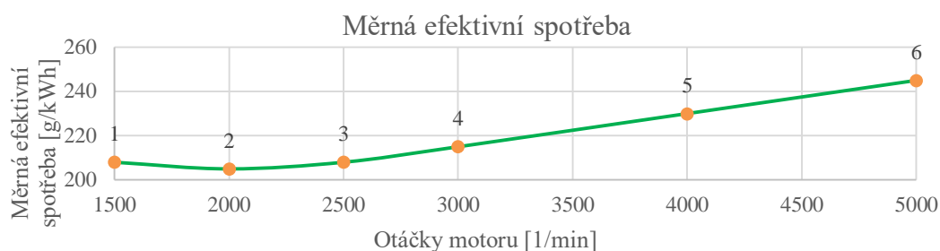
Obr. 40 Zvolený průběh měrné efektivní spotřeby paliva
