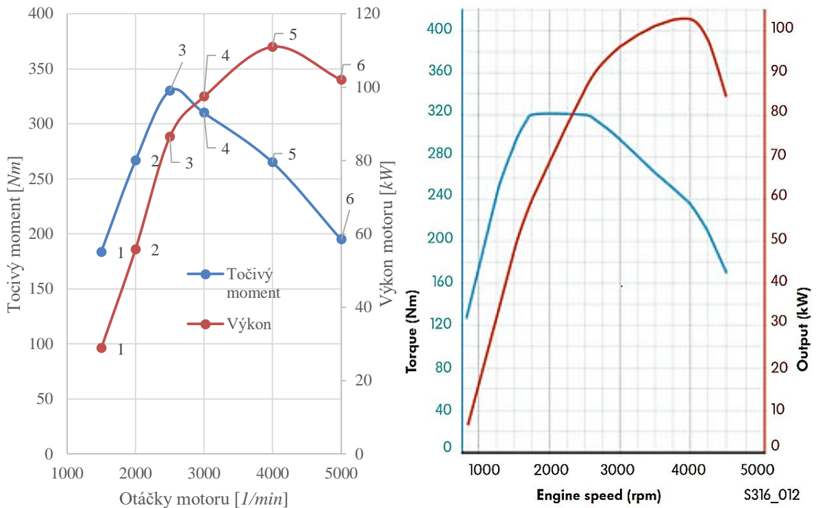
Obr. 46 Odhadovaná výkonová charakteristika motoru 2.0TDI vybaveného turbodmychadlem GT2052 v porovnání s původní
