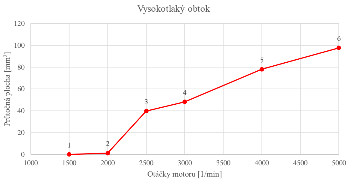
Obr. 54 Průtočná plocha vysokotlakého obtokového ventilu v závislosti na otáčkách motoru
