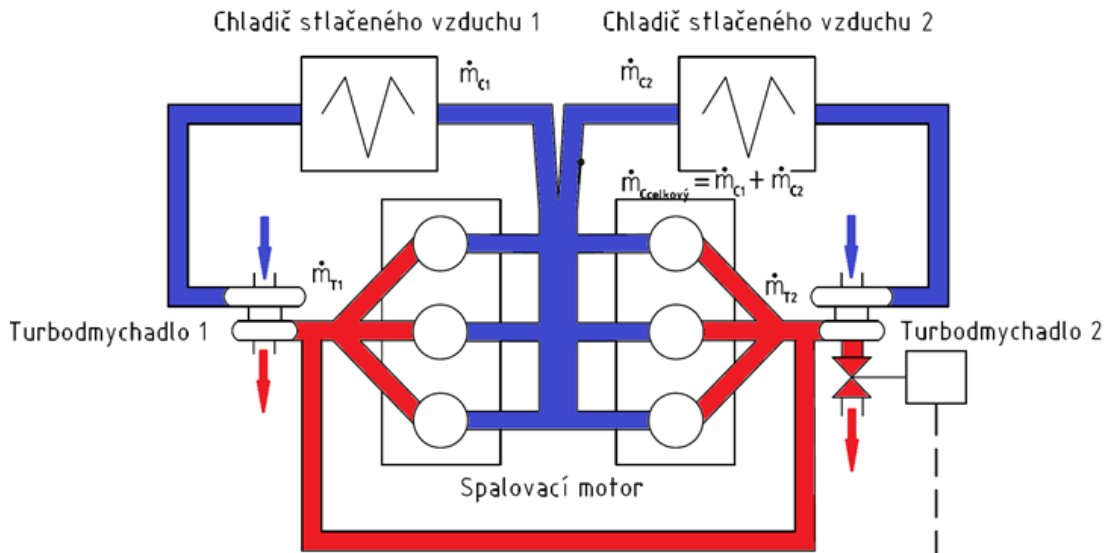
Obr. 22 Paralelní zapojení turbodmychadel, vysoké otáčky motoru [1] – upraveno
