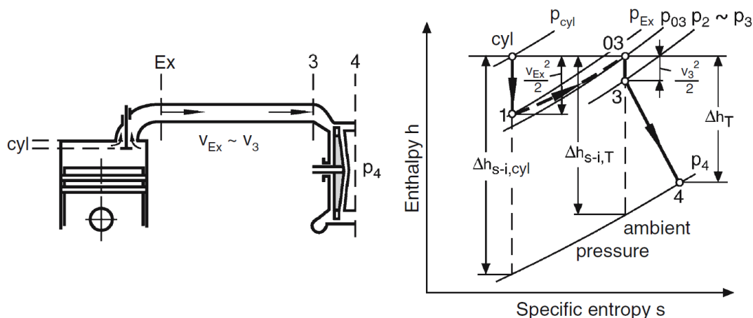
Obr. 9 Schéma pulzního přeplňování a h-s diagram děje [1]
