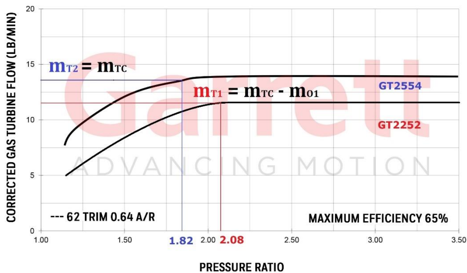
Obr. 27 Znáznornění pracovních bodů v oblasti řízení pomocí obtoku [4] – upraveno
