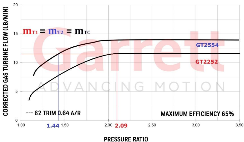
Obr. 24 Znáznornění pracovních bodů turbín [4] – upraveno
