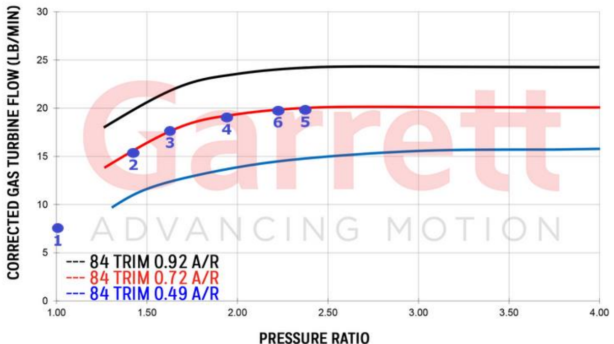
Obr. 64 Turbínová charakteristika nízkotlakého turbodmychadla se zakreslenými pracovními body [4] – upraveno
