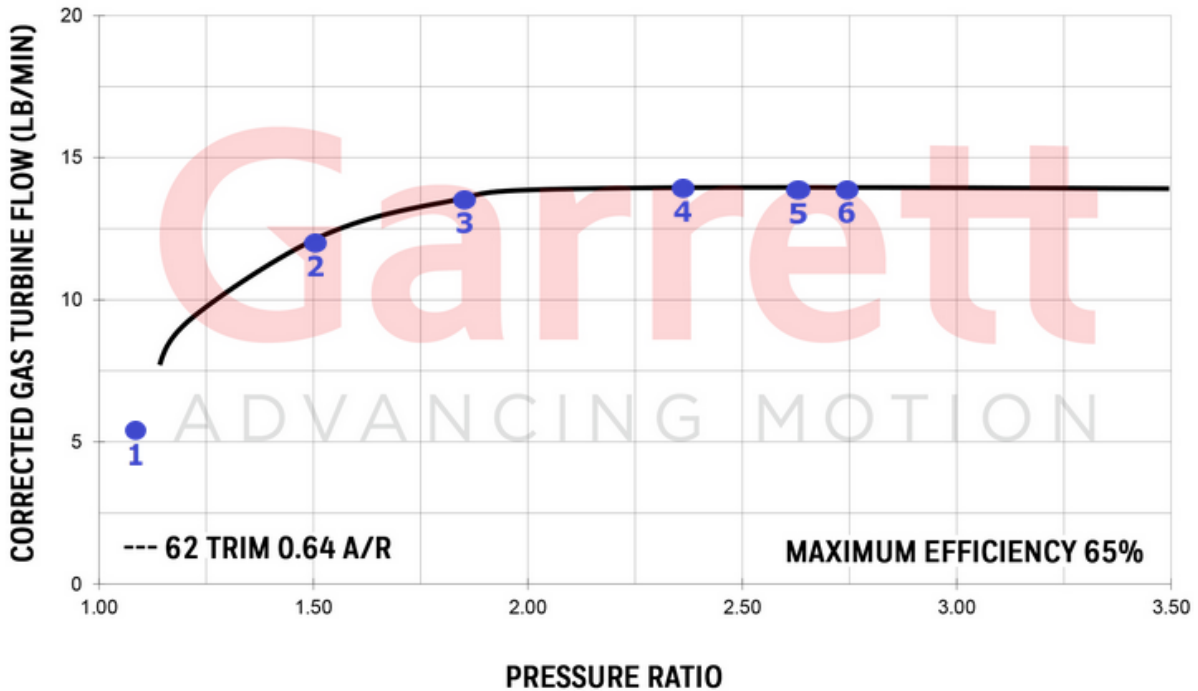
Obr. 52 Pracovní body zakreslené v charakteristice nízkotlaké turbíny [4] - upraveno
