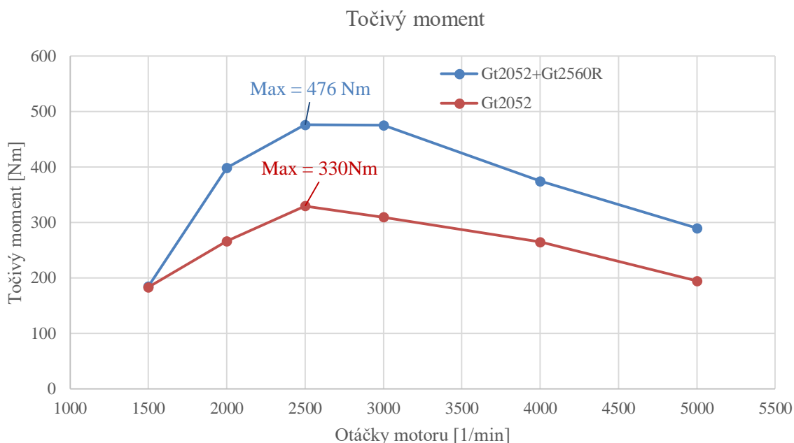
Obr. 57 Porovnání točivého momentu jednostupňově a dvoustupňově přeplňovaného motoru
