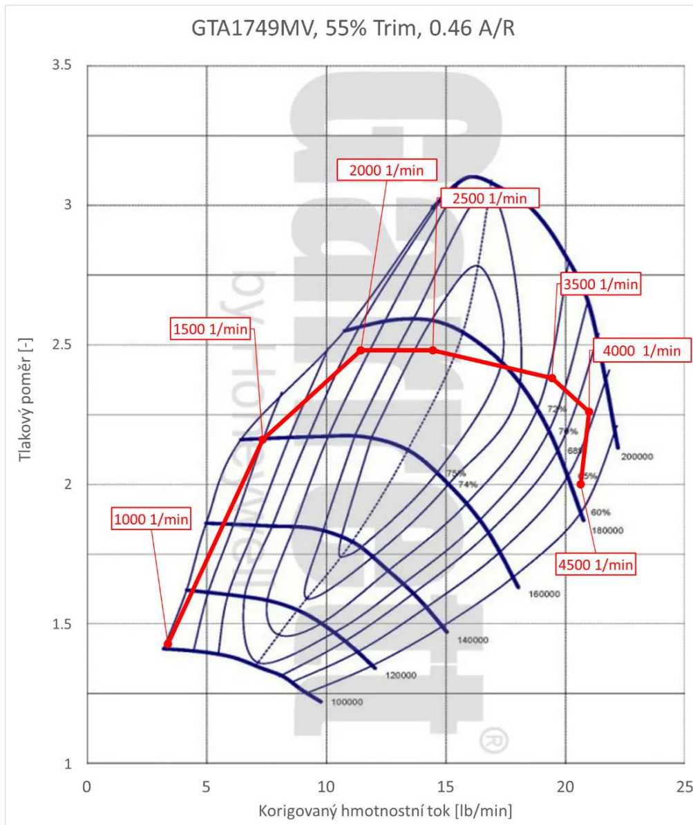
Obr. 36 Pracovní body kompresoru turbodmychadla Garrett GTA1749VM ve spolupráci s motorem EA188 BKD [19] – upraveno
