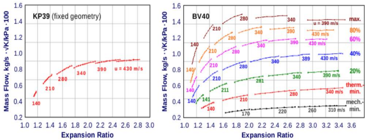
Obr. 17 Porovnání turbínových map [10]
