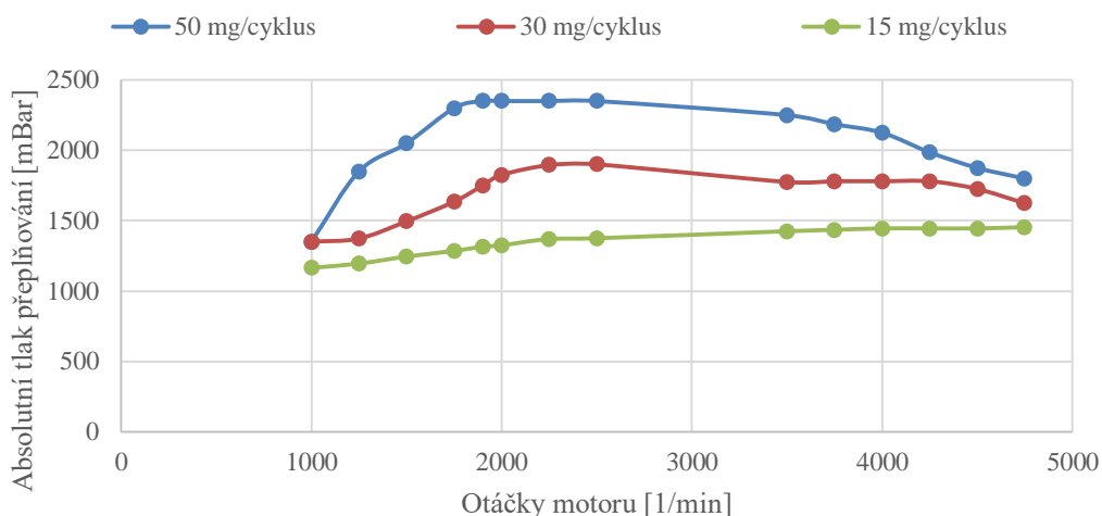
Obr. 35 Znáornění požadavku hodnoty plnicího tlaku v závislosti na množství paliva [zdroj: řídicí jednotka motoru Bosch EDC16 č. 0281011786, č. sw: 375893]
