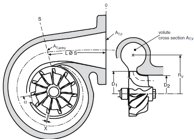
Obr. 11 Znáornění A/R parametru lopátkového stroje
