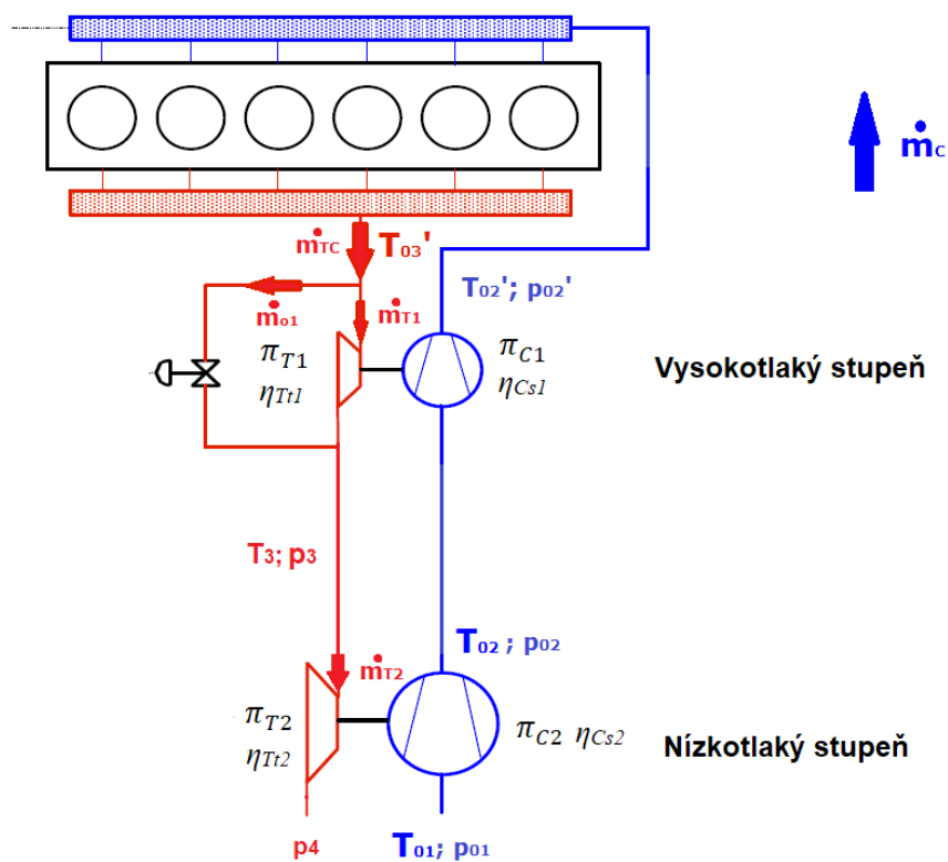
Obr. 26 Řízené sériové zapojení turbodmychadel [12] – upraveno
