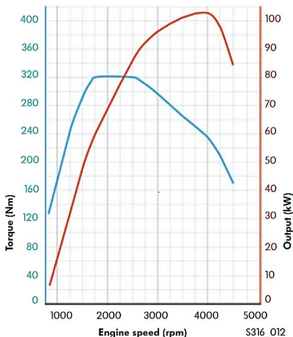
Obr. 34 Průběh výkonu a točivého momentu motoru 2.0TDI BKD [17]
