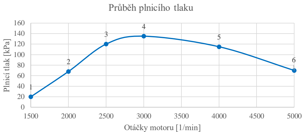
Obr. 38 Určený průběh relativní hodnoty plicního tlaku
