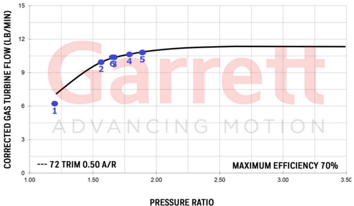
Obr. 63 Turbínová charakteristika vysokotlakého turbodmychadla se zakreslenými pracovními body [4] – upraveno
