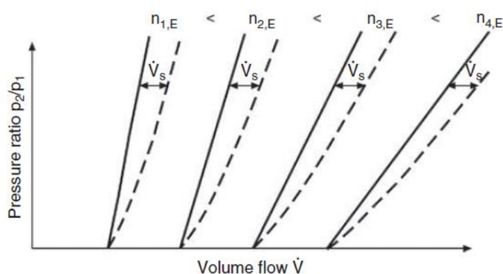
Obr. 7 Pracovní charakteristiky čtyřdobého motoru [1]
