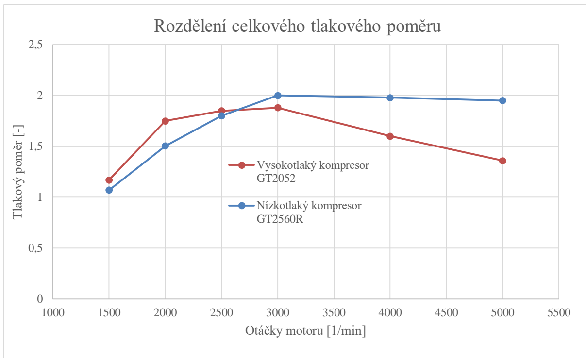
Obr. 53 Rozdělení celkového tlakového poměru
