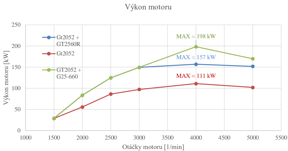
Obr. 67 Průběh výkonu s turbodmychadly, porovnání jednotlivých variant
