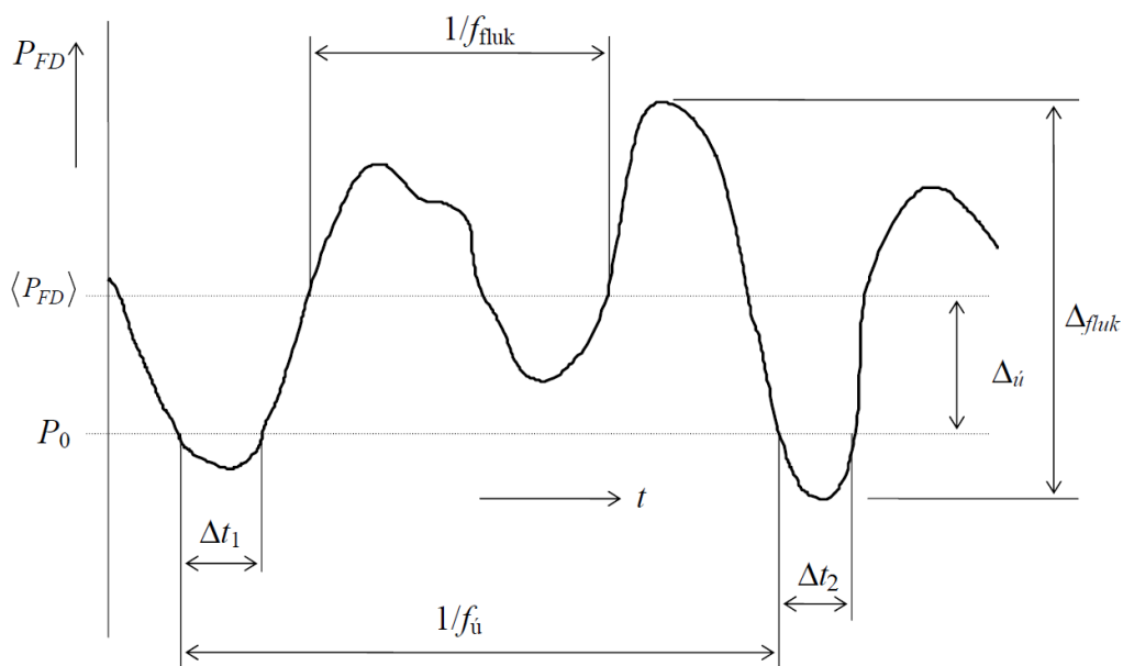
Obrázok 1.3: parametre fluktuácií a únikov [1] ( P_{FD} – optický výkon na fotodióde prijímača, P_0 – citlivosť prijímača, f_{flukt} – frekvencia fluktuácií, f_{\dot{u}} – frekvencia únikov, \Delta_{fluk} – dynamika fluktuácií, \Delta_{\dot{u}} – hĺbka únikov, t – čas, \Delta t_i – časové intervaly únikov)
