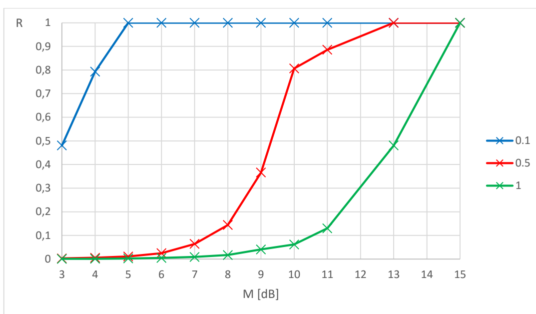
Obrázok 3.4: výsledky simulácie (bez vyrovnávacej pamäti)
