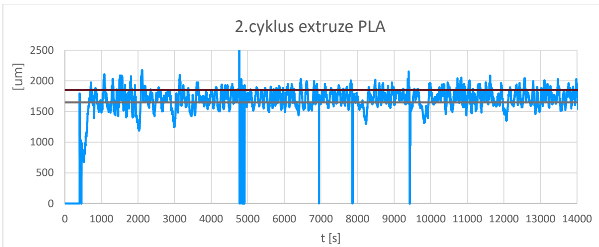
Obr. 5-1 Průběh průměru filamentu při extruzi v druhém cyklu
