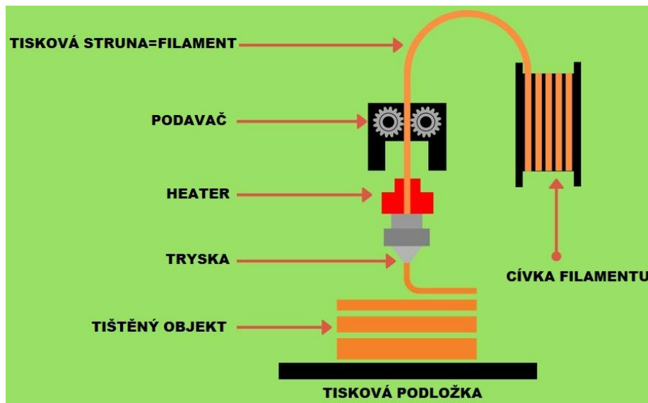
Obr. 2-1 Schéma technologie FDM [7]
