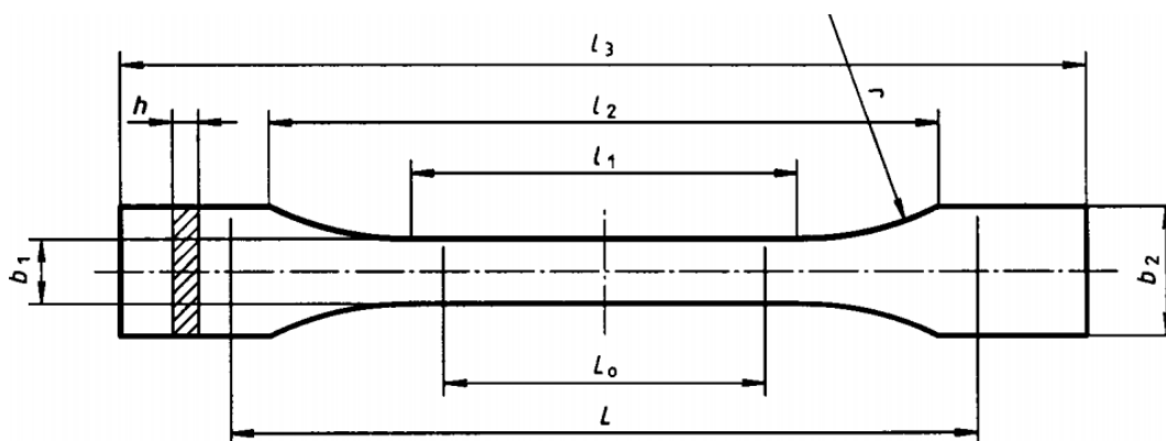
Obr. 4-5 Rozměry tištěného zkušebního tělesa
