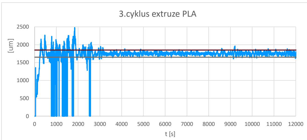
Obr. 5-2 Průběh průměru filamentu při extruzi ve třetím cyklu
