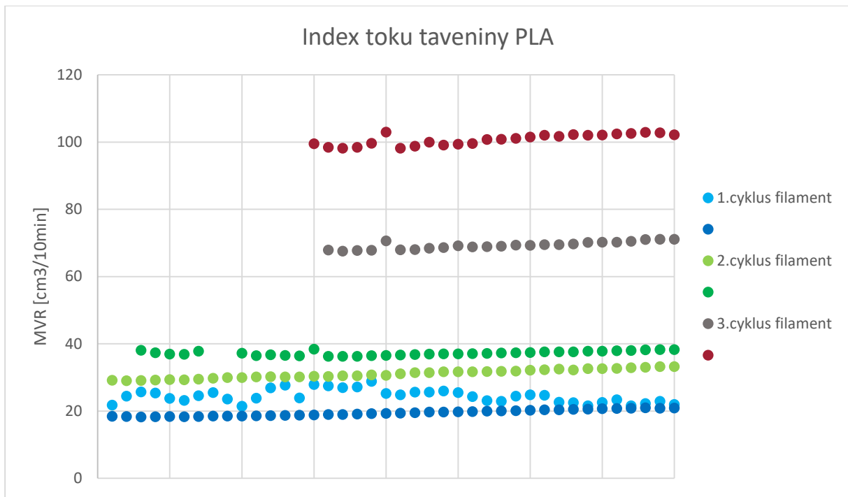
Obr. 5-8 Graf indexu toku taveniny
