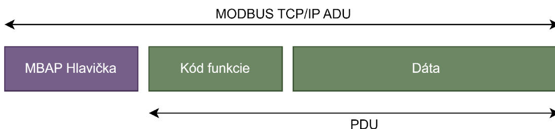
Obr. 3.3: MODBUS Žiadosť/Odpoveď cez TCP/IP [4]
