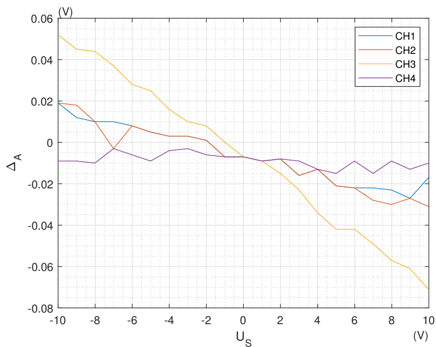
Obr. F.1: Absolútna chyba merania analógových vstupov
