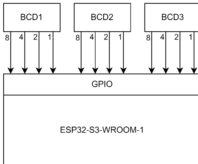
Obr. 5.8: Zjednodušená bloková schéma pripojenia BCD prepínačov
