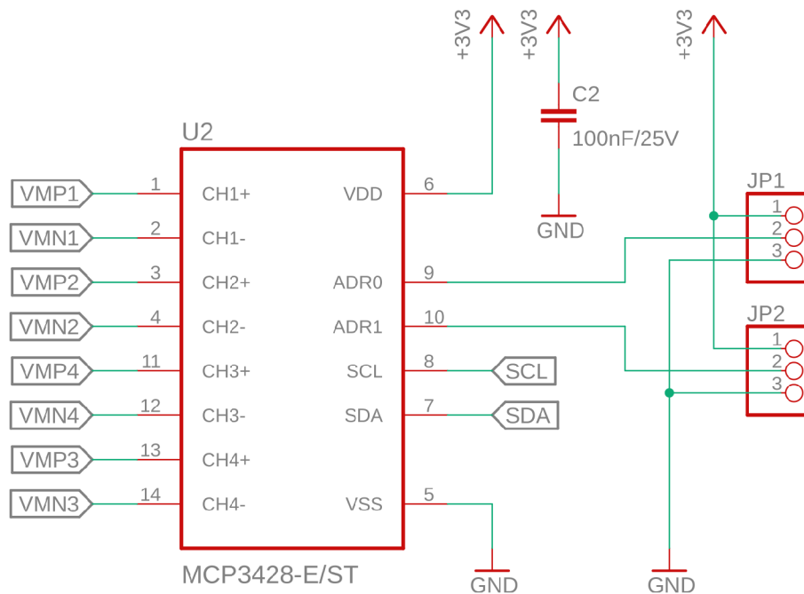
Obr. 5.19: Schéma zapojenia ADC
