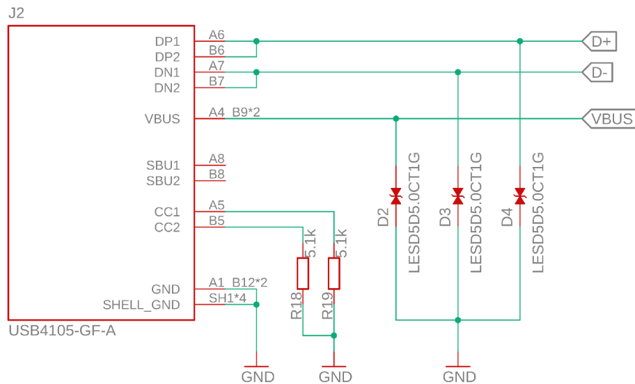
Obr. 5.7: Schéma zapojenia USB rozhrania
