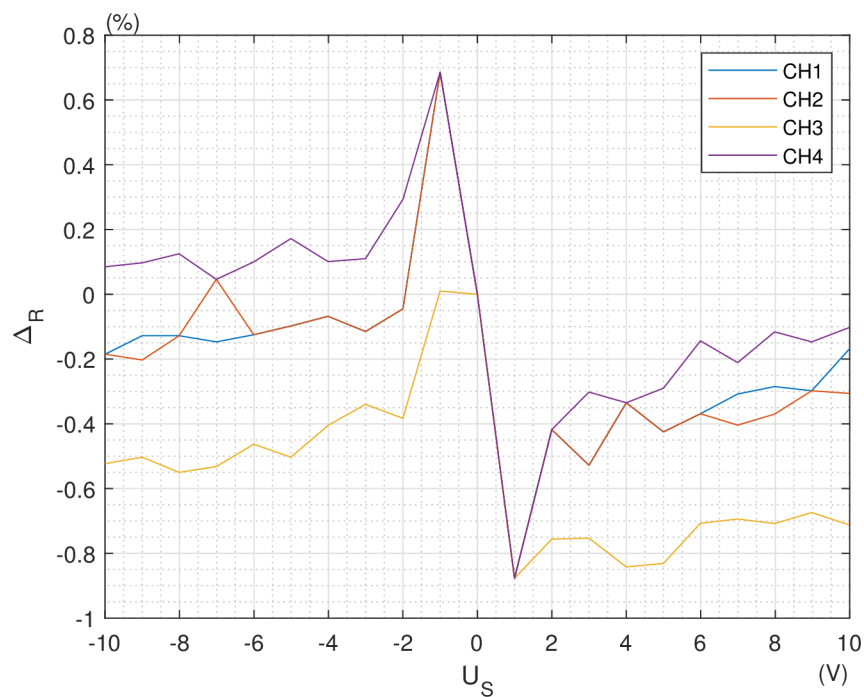
Obr. F.2: Relatívna chyba merania analógových vstupov
