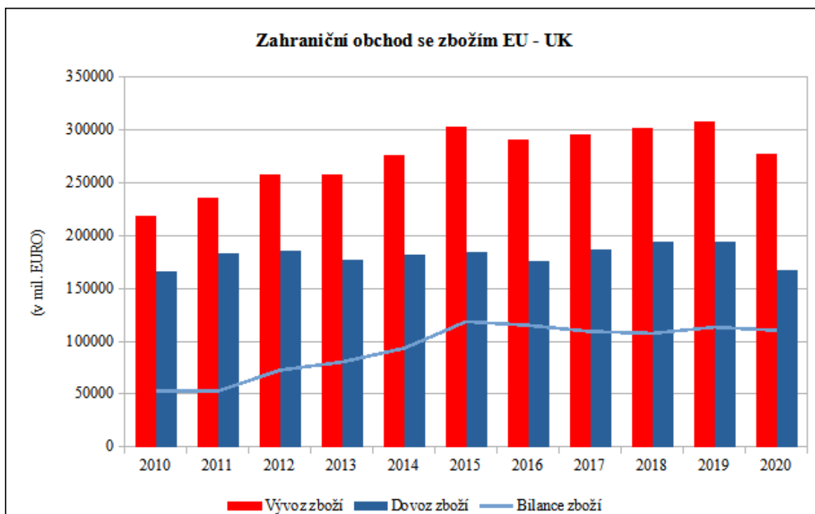
Obrázek 6: Graf zahraničního obchodu se zbožím EU – UK
