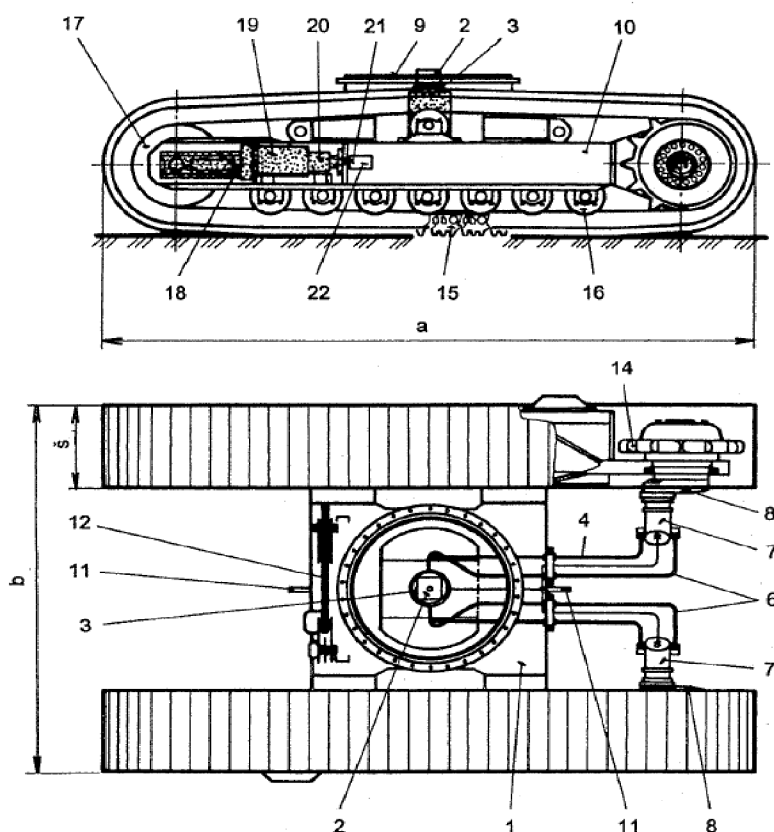
Hlavní části a uspořádání pásových podvozků: 1 – rám podvozku, 2 – hydraulický převaděč, 3 – pouzdro, 4 – tlakové či odpadové potrubí pro jezdové hydromotory, 6 – odpadové (tlakové) potrubí, 7 – rotační jezdové hydromotory, 8 – koncové převody, 9 – nosný věnec velkorozměrového ložiska, 10 – podélný nosič pásů podvozku, 11 – tažné závěsy, 12 – opěrná deska, 14 – hnací turasové kolo, 15 – články řetězu, 16 – nosné jezdové kladky, 17 – vodící napínací kolo, 18 – třmen napínacího ústrojí, 19 – válcový tlumič, 20 – prostor pro plnění tuku, 21 – tuková plnicí maznička, 22 – uzávěr.
