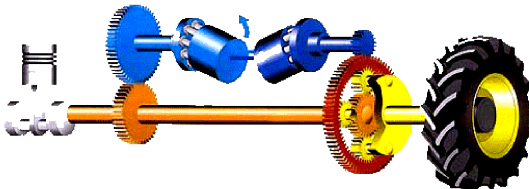
Obr. 11 Schéma znázorňující princip funkce CVT převodovky [2]
