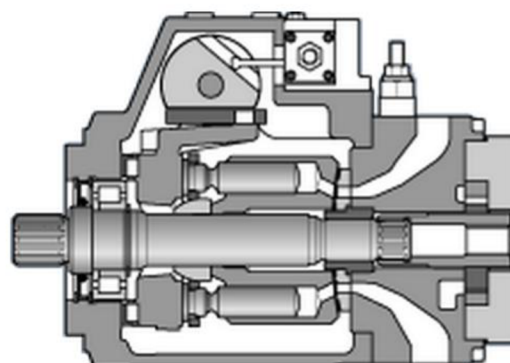
Obr. 21 Hydrogenerátor Bosch Rexroth A4VG/32
