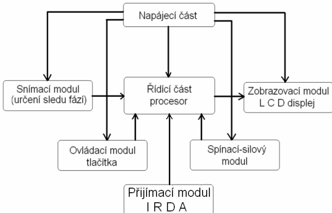
Obr.4.4. Blokové schéma fázovacího modulu
