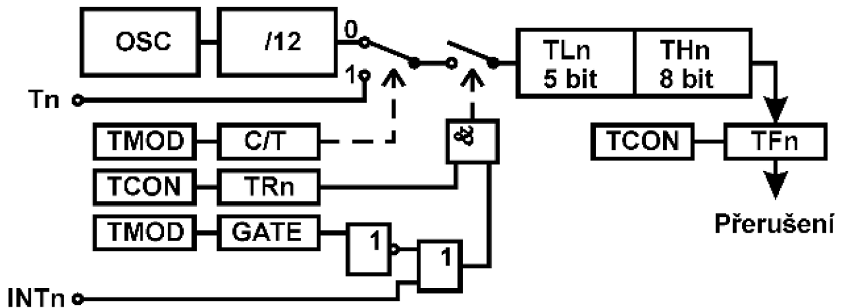
Obr 4.3. Blokové schéma čítače / časovače a v módu 0
