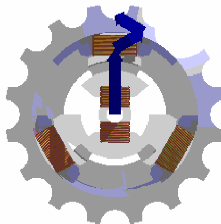
Obr.2.2. Řez synchronního motoru
