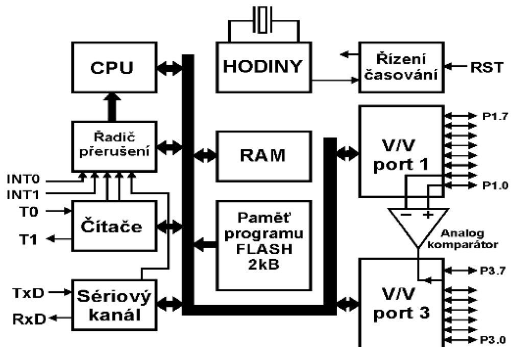
Blokové schéma procesoru AT89C2051
