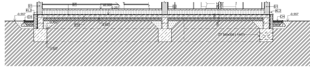
ŘEZ B-B
