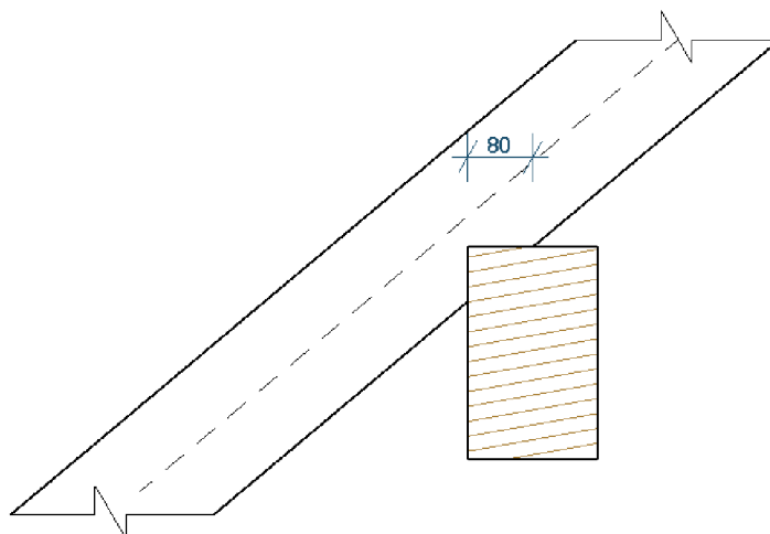
Obrázek 34 Osedlání krokve na vaznici
