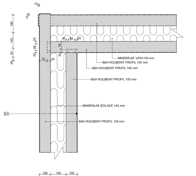
VARIANTA SC - ROUBENÍ S VLOŽENOU IZOLACÍ
