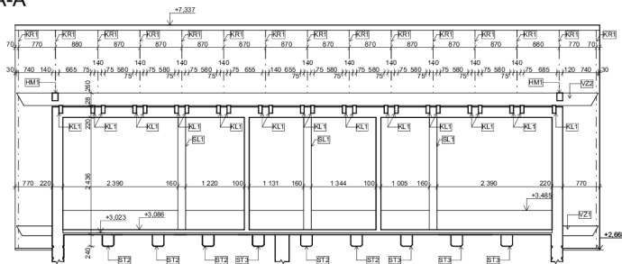
ŘEZ A-A
