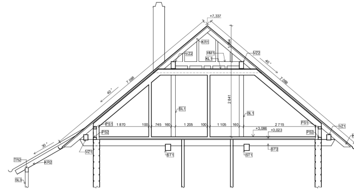
ŘEZ B-B
