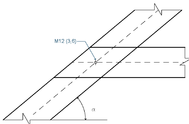
Obrázek 31 Provedení spoje kleštiny – krovky
