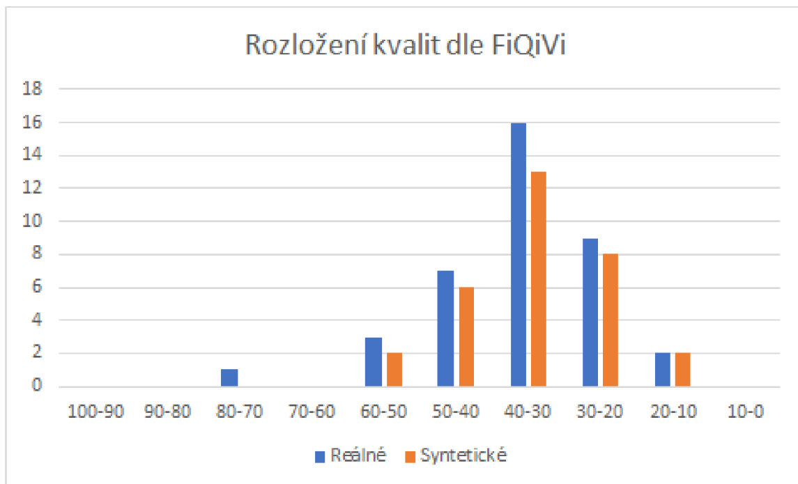
Obrázek 7.2: Histogram rozložení reálných a syntetických otisků dle FiQVi seskupených po 10-ti procentech.
