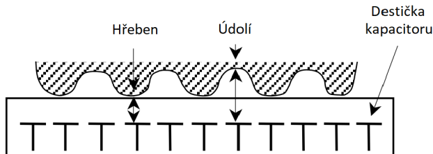
Obrázek 2.6: Schéma kapacitního senzoru z [26].
