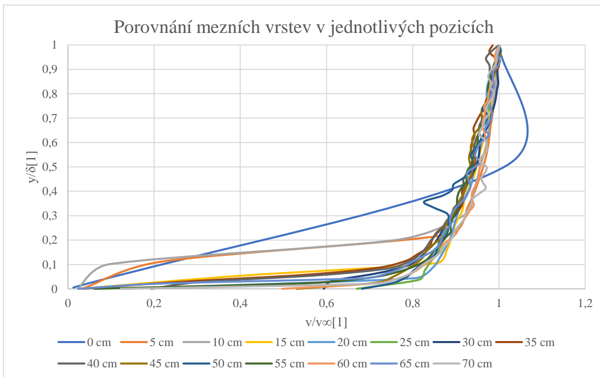
Graf 2: Porovnání mezních vrstev
