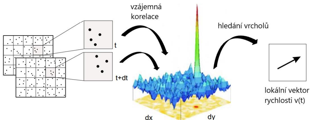
Obr. 9: Vyhodnocení záznamu pomocí vzájemné korelace [7]
