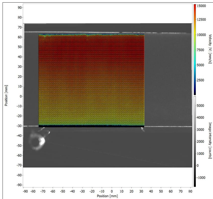
Obr. P 1. 6: Průměrné rychlostní pole na konci obtékané desky
