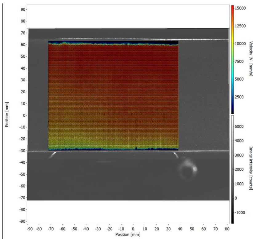
Obr. P 1. 4 Průměrné rychlostní pole ve středním úseku obtékané desky
