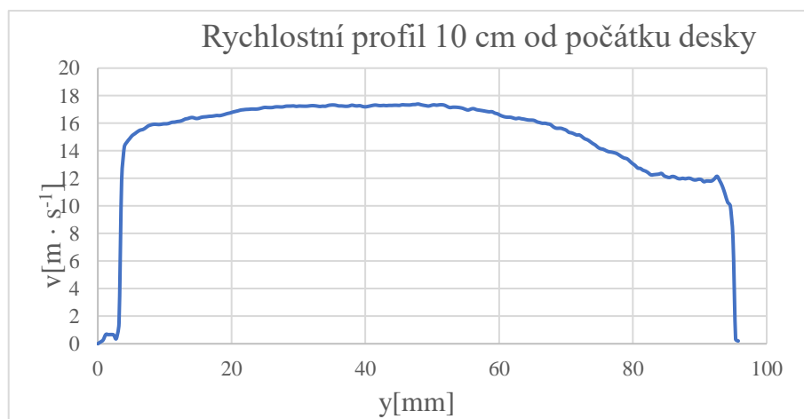
Graf P 2. 3: Rychlostní profil 10 cm od počátku
