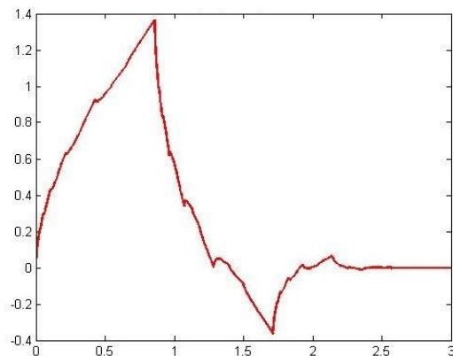
Obrázok 6: Vlnka db4 [16]
