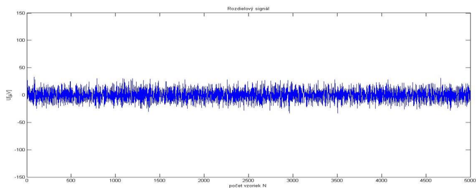
Obrázok 10: Rozdielový signál
