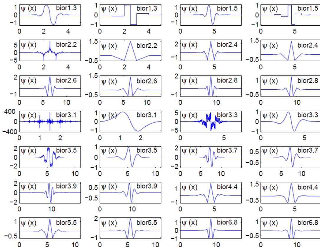
Obrázok 7: Biortogonálne vlnky [18]
