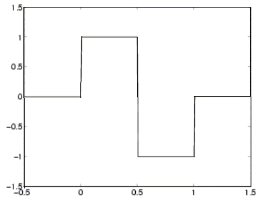
Obrázok 5: Haarova vlnka [16]
