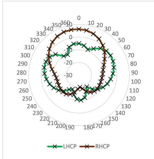
Obr. 21 Vyzářovací charakteristika antény v rovině xz . Simulovaná LHCP (zeleně) a RHCP (hnědě).
