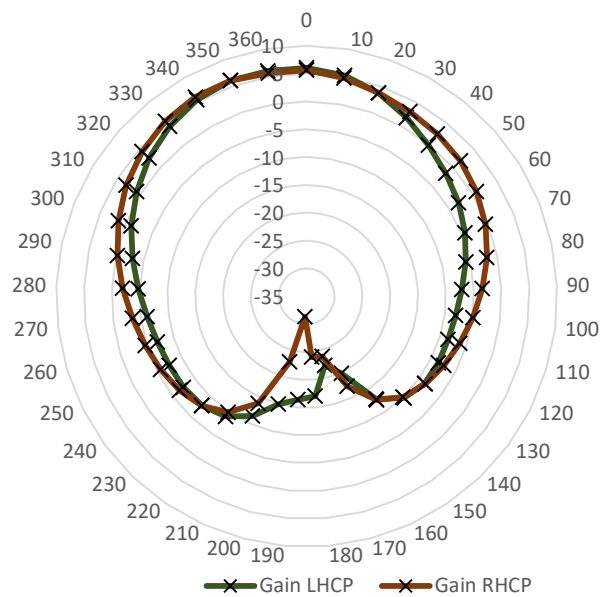
Obr. 16 Vyzařovací charakteristika flíčkové antény v rovině yz . Simulovaná LHCP (zeleně) a RHCP (hnědě).
