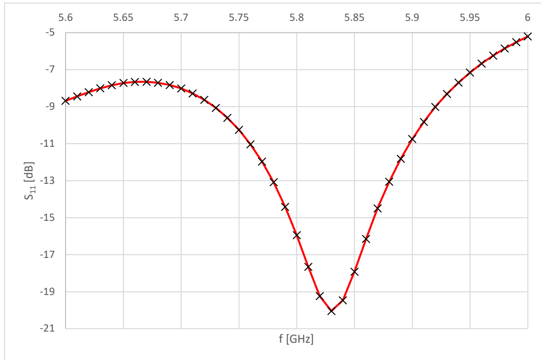
Obr. 13 Kmitočtový průběh velikosti činitele odrazu na vstupu kruhově polarizované flíčkové antény. Výsledek simulace numerického modelu.
