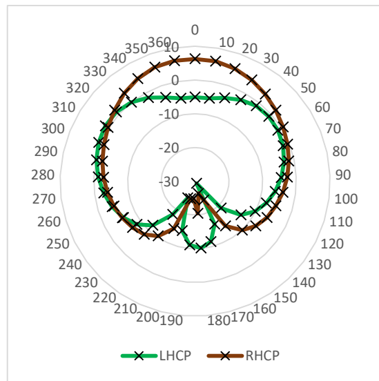
Obr. 22 Vyzářovací charakteristika antény v rovině yz . Simulovaná LHCP (zeleně) a RHCP (hnědě).
