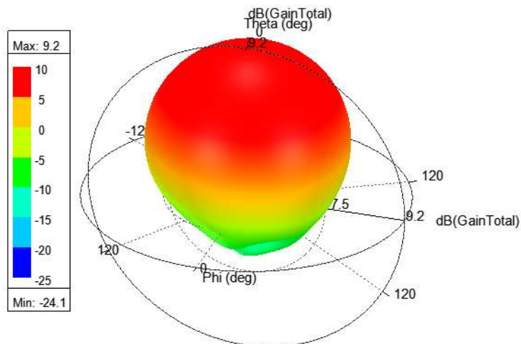
Obr. 29 3D směrová charakteristika kruhově polarizované flíčkové antény. Simulováno v ANSYS HFSS.
