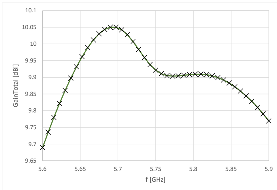
Obr. 9 Kmitočtový průběh celkového zisku. Výsledek simulace numerického modelu.
