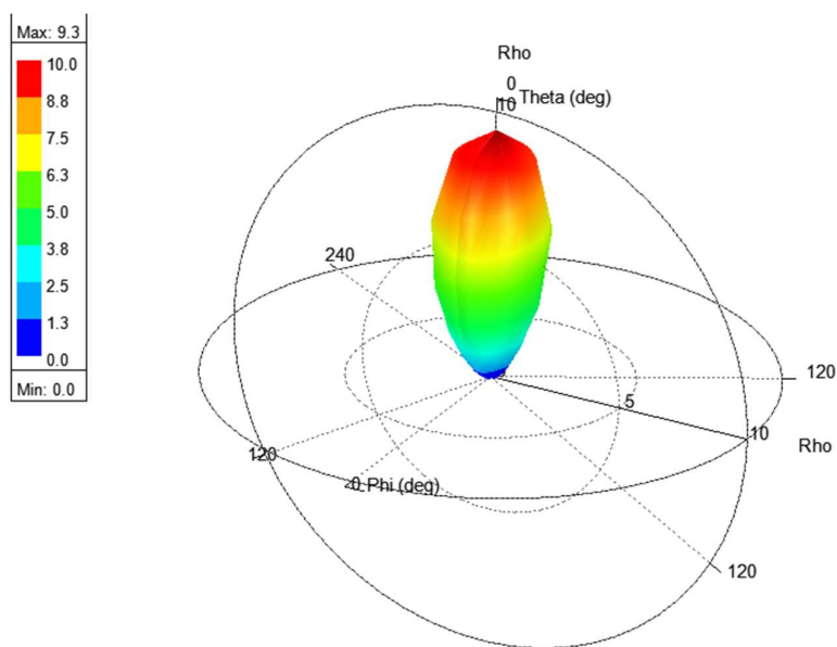
Obr. 10 3D směrová charakteristika simulované antény. Výsledek simulace numerického modelu.
