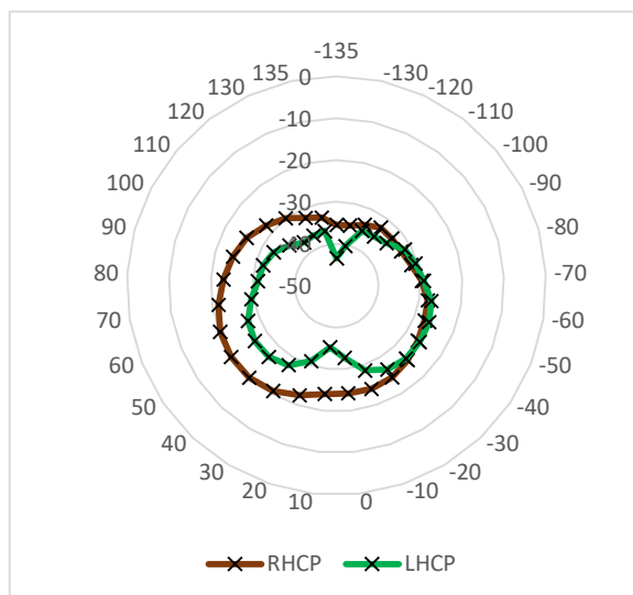
Obr. 46 Vyzařovací charakteristiky planární antény v rovině xz Změřená LHCP (zeleně) a RHCP (hnědě).
