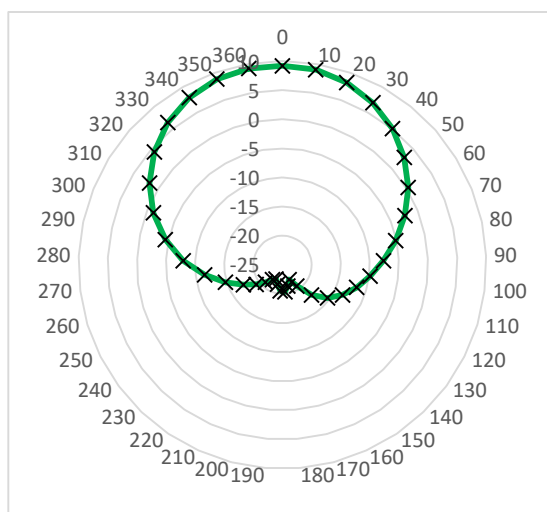
Obr. 27 Vyzářovací charakteristika kruhově polarizované flíčkové antény ve směru vyzářování LHCP, v rovině xz .
