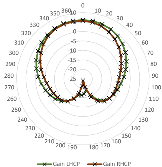
Obr. 15 Vyzařovací charakteristika flíčkové antény v rovině xz . Simulovaná LHCP (zeleně) a RHCP (hnědě).
