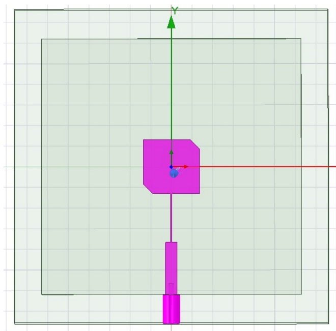
Obr. 12 Numerický model pravotočivě polarizované flíčkové antény.
