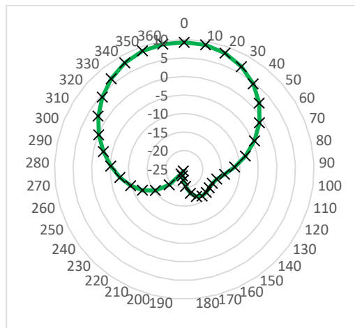
Obr. 28 Vyzařovací charakteristika kruhově polarizované flíčkové antény ve směru vyzařování LHCP, v rovině yz.
