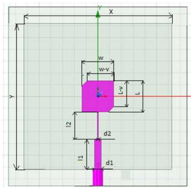
Obr. 11 Numerický model levotočivě polarizované flíčkové antény.
