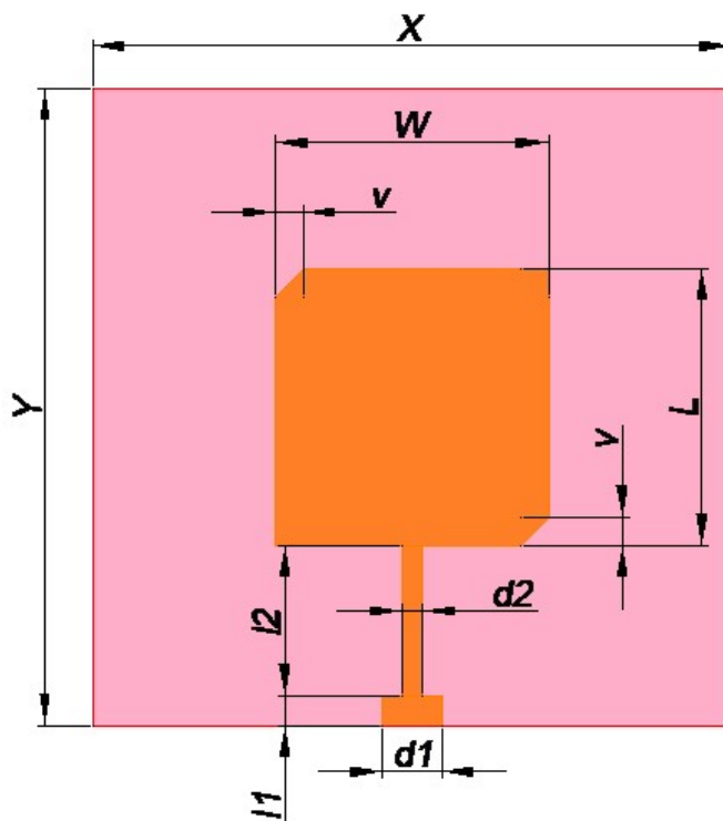
Obr. 24 Numerický model levotočivě polarizované flíčkové antény.
