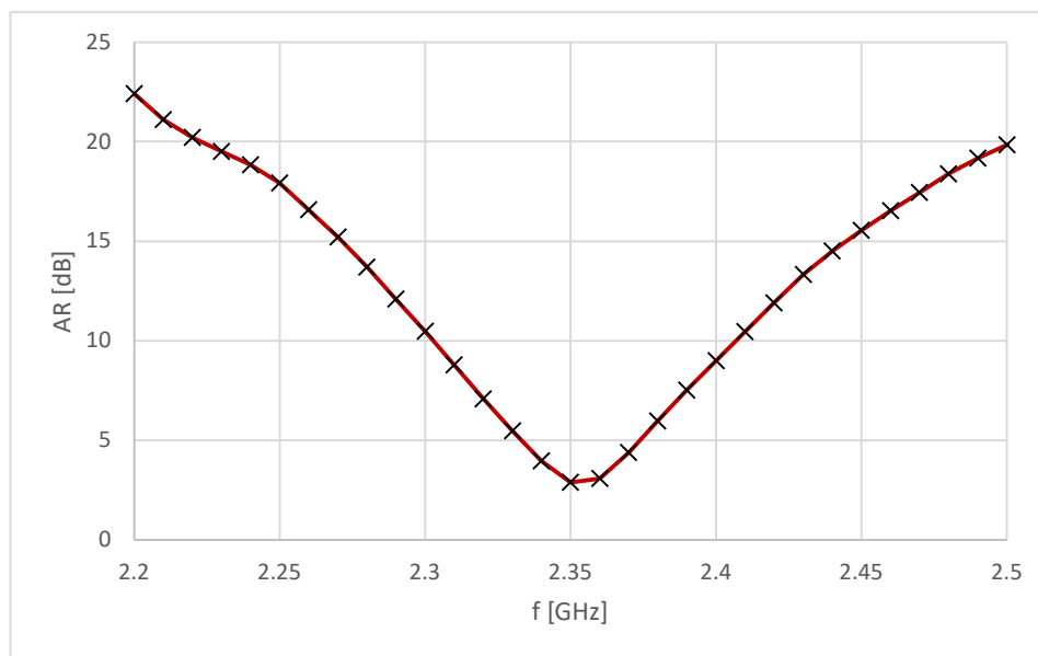
Obr. 41 Kmitočtový průběh osového poměru kruhově polarizované flíčkové antény. Výsledek změřeného průběhu.
