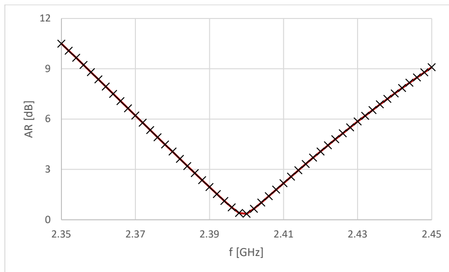
Obr. 26 Kmitočtový průběh osového poměru kruhově polarizované flíčkové antény. Výsledek simulace numerického modelu.
