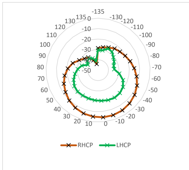
Obr. 42 Vyzařovací charakteristiky flíčkové antény v rovině xz Změřená LHCP (zeleně) a RHCP (hnědě).
