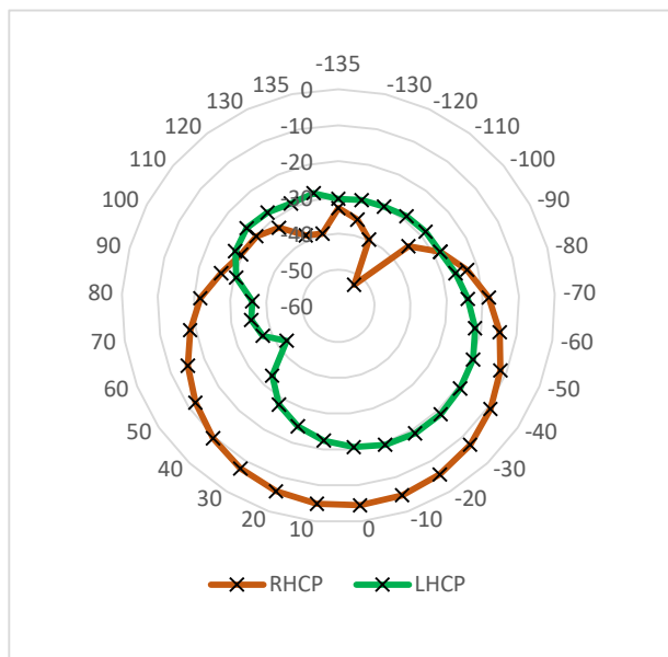
Obr. 43 Vyzařovací charakteristiky flíčkové antény v rovině yz Změřená LHCP (zeleně) a RHCP (hnědě).
