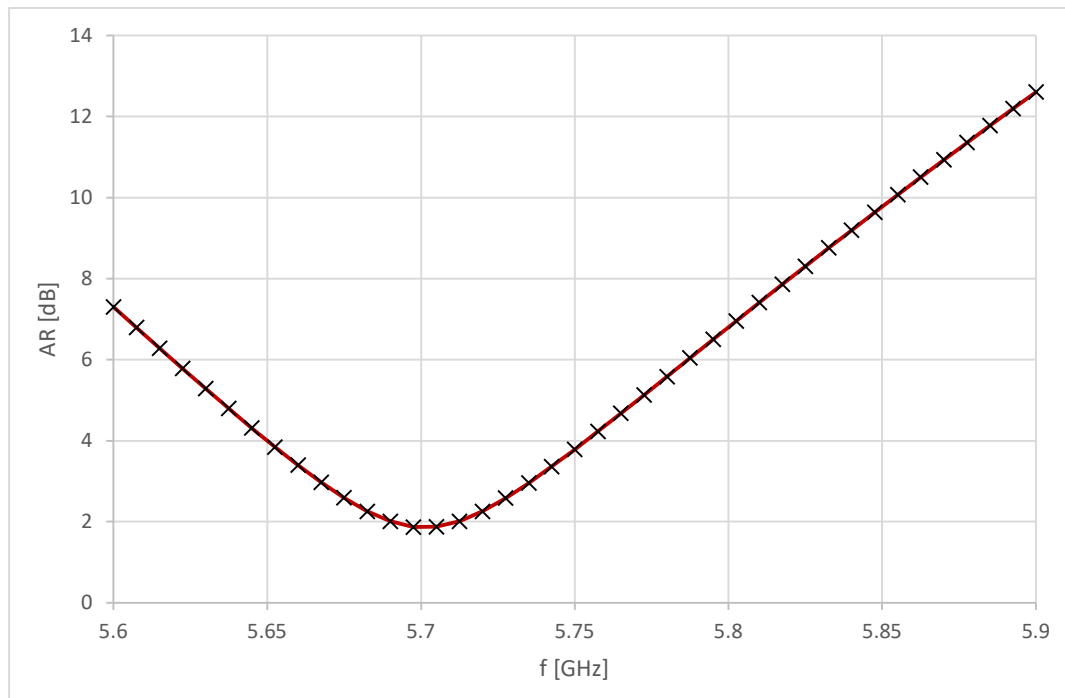
Obr. 14 Kmitočtový průběh osového poměru kruhově polarizované fličkové antény. Výsledek simulace numerického modelu.
