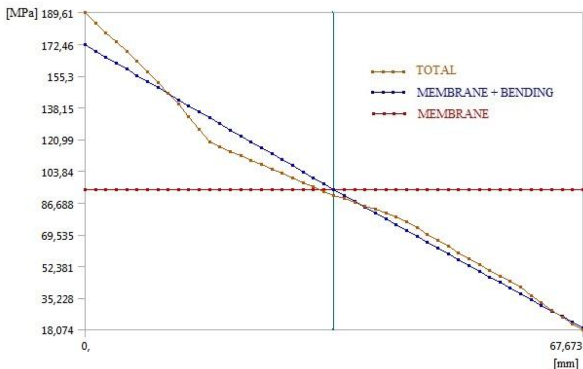
Obr. 4.4.3.1 – Linearizované napětí pro provozní podmínky
