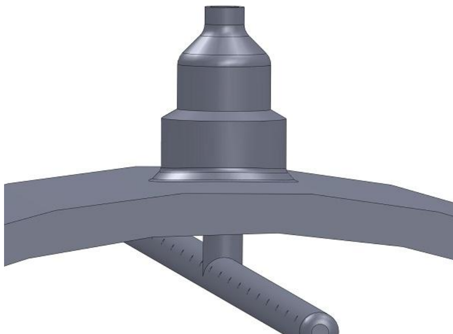
Obr. 4.4.1 – Model hrdla B4 s integrovanou trubicí Blowdownu
