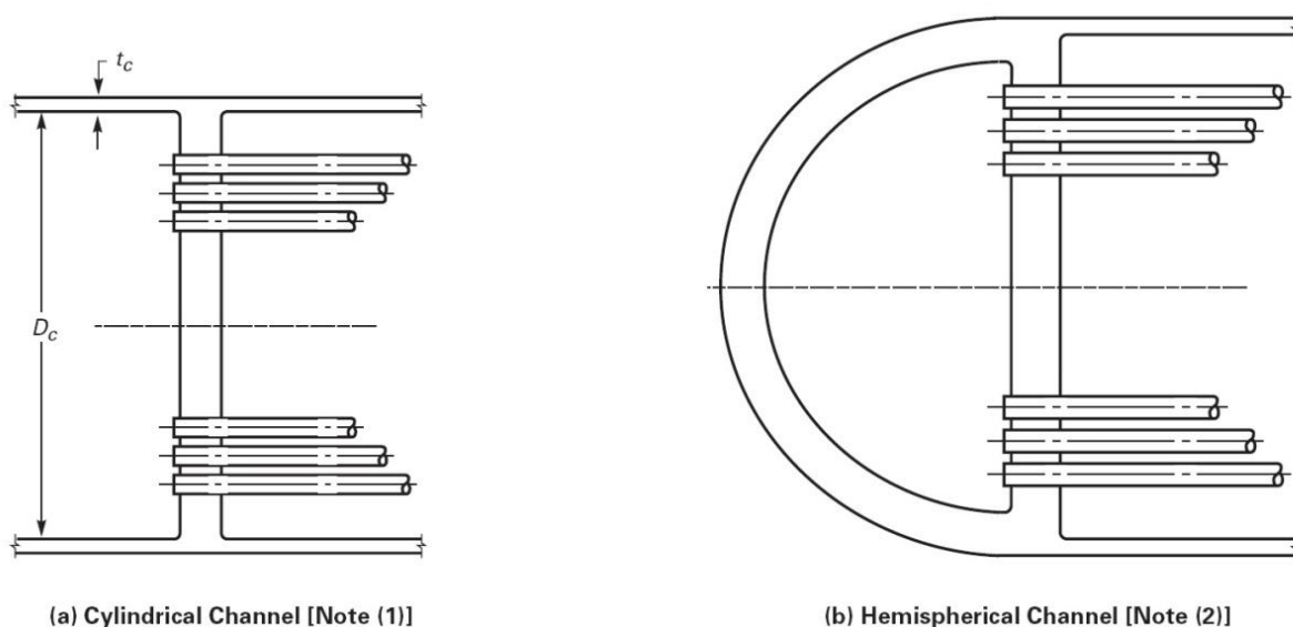
Obr. 3.7.1 – Typy komor [1]
