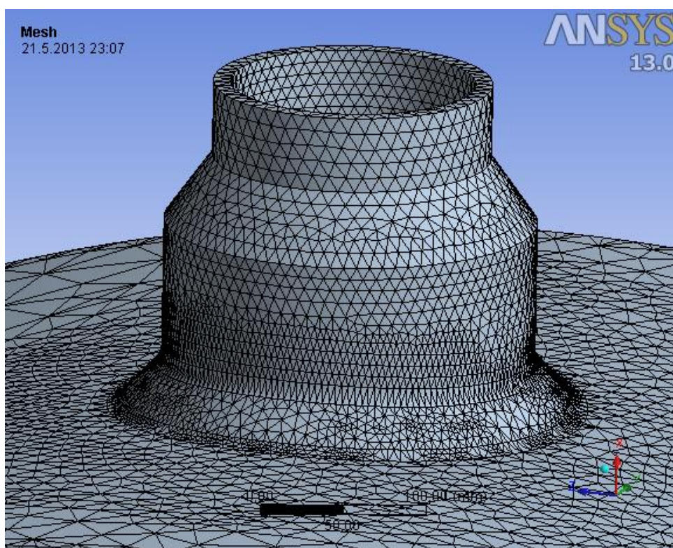
Obr. 4.3.1.1 – Sít' konečných prvků
