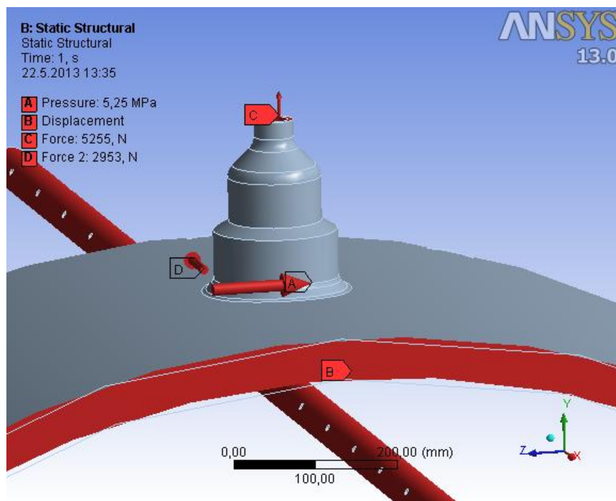
Obr. 4.4.1.2 – Okrajové podmínky
