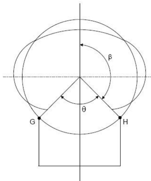
Obr. 3.6.4.1 – Maximální obvodový ohybový moment v místě podpory [2]
