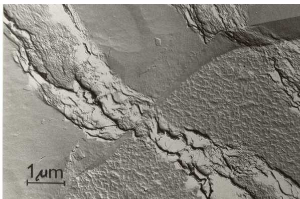
Obr. 2.2.1.1 – Mikrotrhlina – přechod přes hranici zrna [10]
