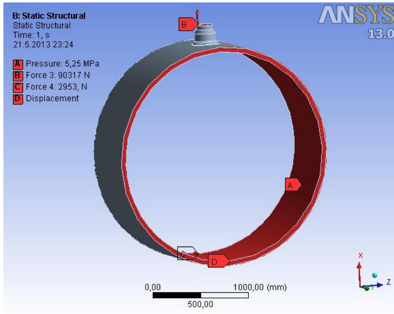
Obr. 4.3.1.2 – Okrajové podmínky
