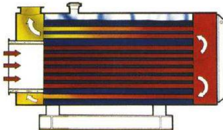
Obr. 2.1.2.1 – Schéma dvouchodého kotle na odpadní teplo [1]
