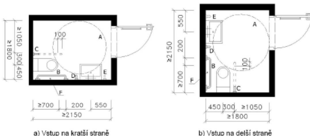
Obrázek 11: Uspořádání kabiny pro invalidy (ČSN 73 4108, 2020)
