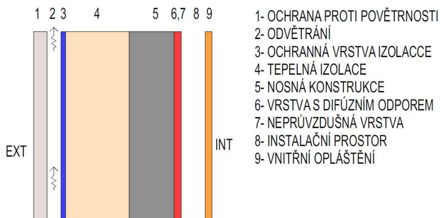
Obrázek 3: Vrstvy pláště (vlastní zpracování)
