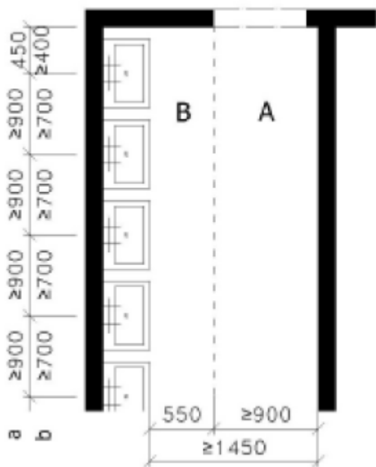
Obrázek 8: Uspořádání umývárny s řadou umyvadel (ČSN 73 4108, 2020)
