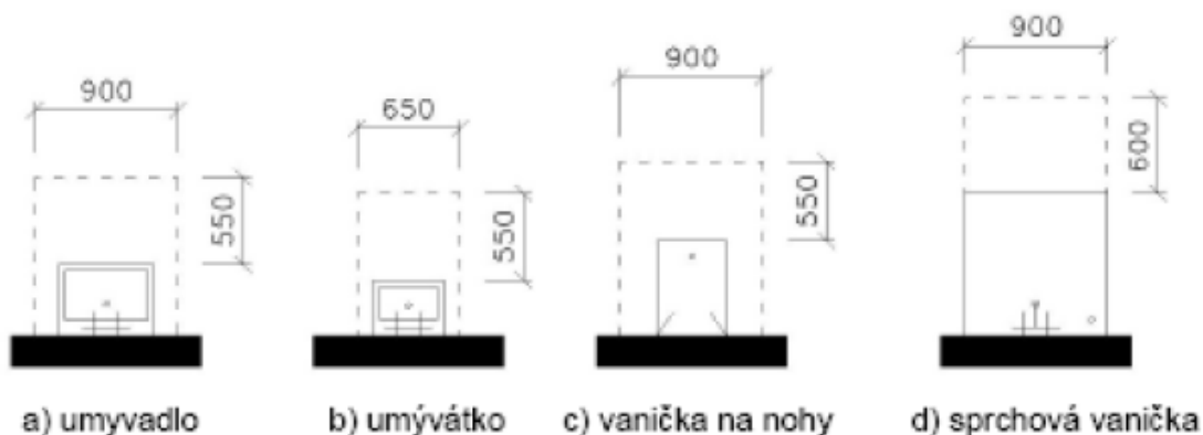
Obrázek 7: Manipulační plocha zařizovacích předmětů (ČSN 73 4108, 2020)
