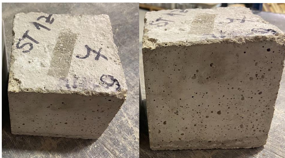
Obr. 29 - Detail povrchu zkušebního tělesa po cyklování suchý mráz+sušárna RECEPTURA 1
