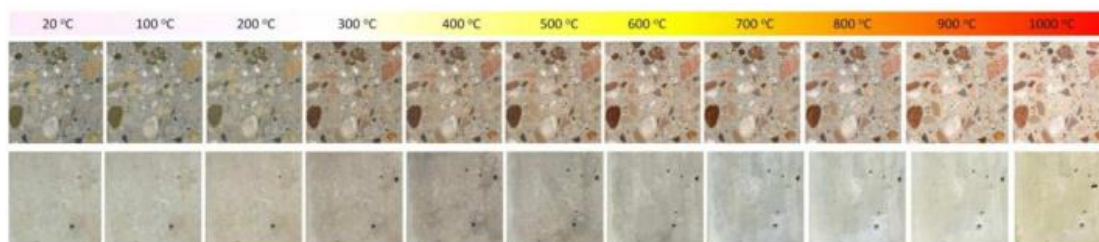
Obr. 6 – Barevné změny betonu při zvyšující se teplotě [27]
