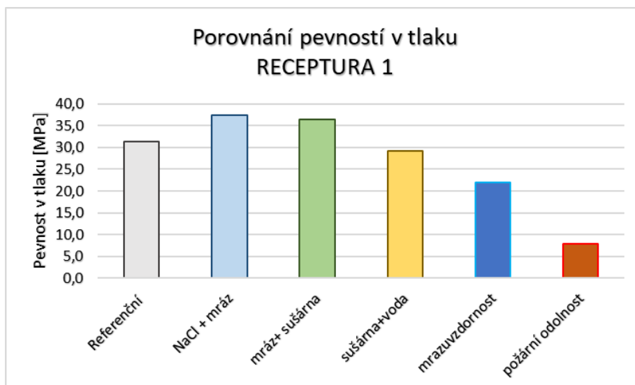
Obr. 31 – Pevnosti v tlaku Receptura 1
