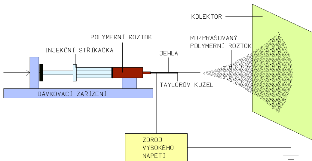
Obrázek 3: Schéma electrosprayingu z jehly [24]
