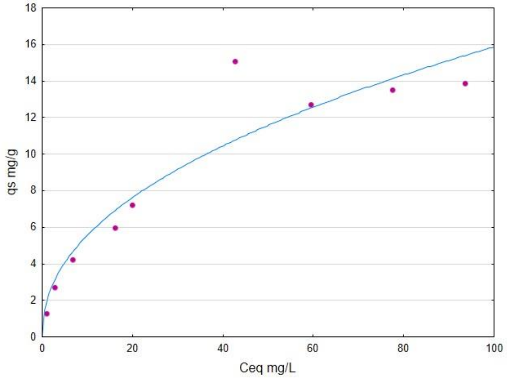
Fig. A4 DCF - BCHTH Freundlich non-linear isotherm
