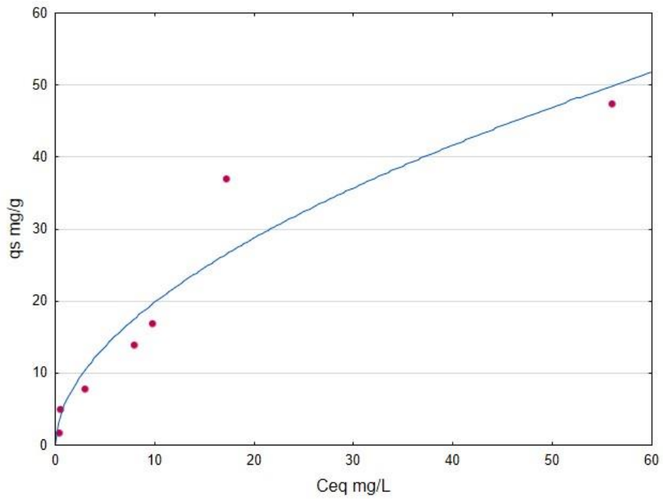
Fig. A24 BTR - BCHSH Freundlich non-linear isotherm
