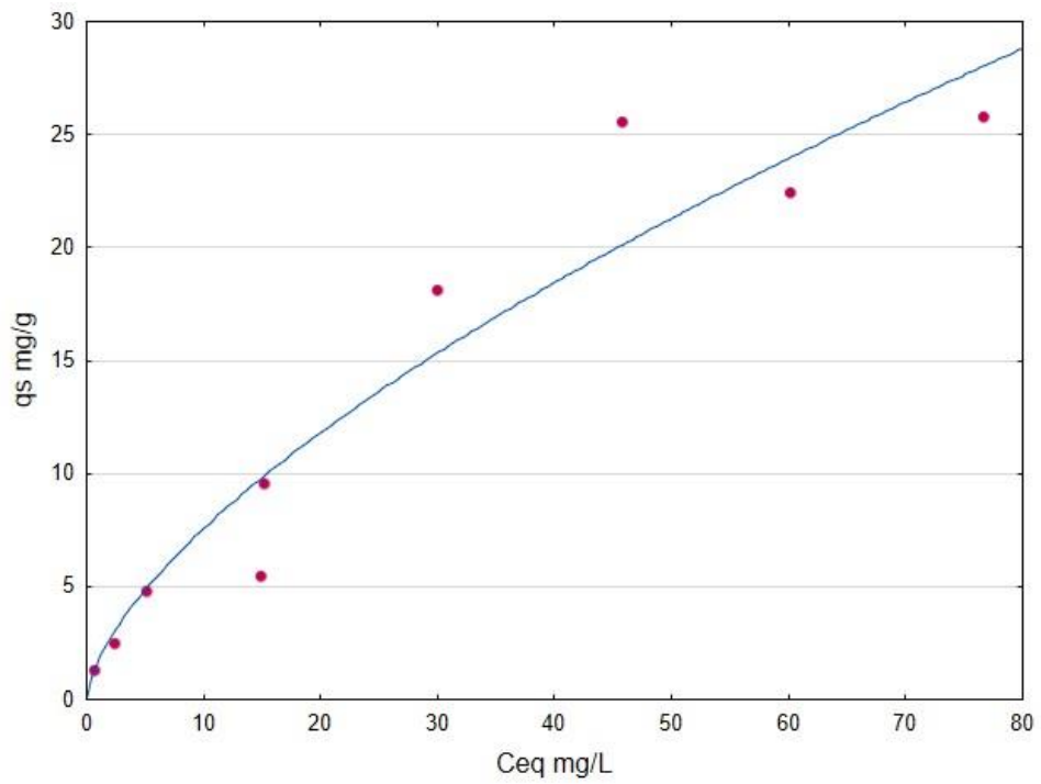
Fig. A20 BTR - BCHTH Freundlich non-linear isotherm
