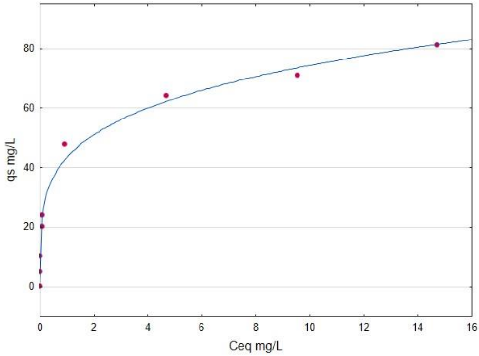
Fig. A16 MTP - BCHSH Freundlich non-linear isotherm
