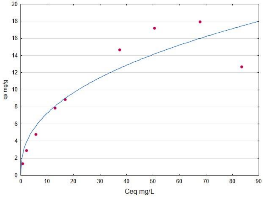
Fig. A10 MTP - BCHTL Freundlich non-linear isotherm
