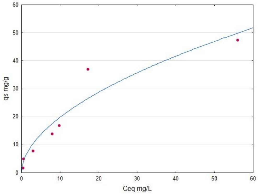
Fig. A22 BTR - BCHSL Freundlich non-linear isotherm
