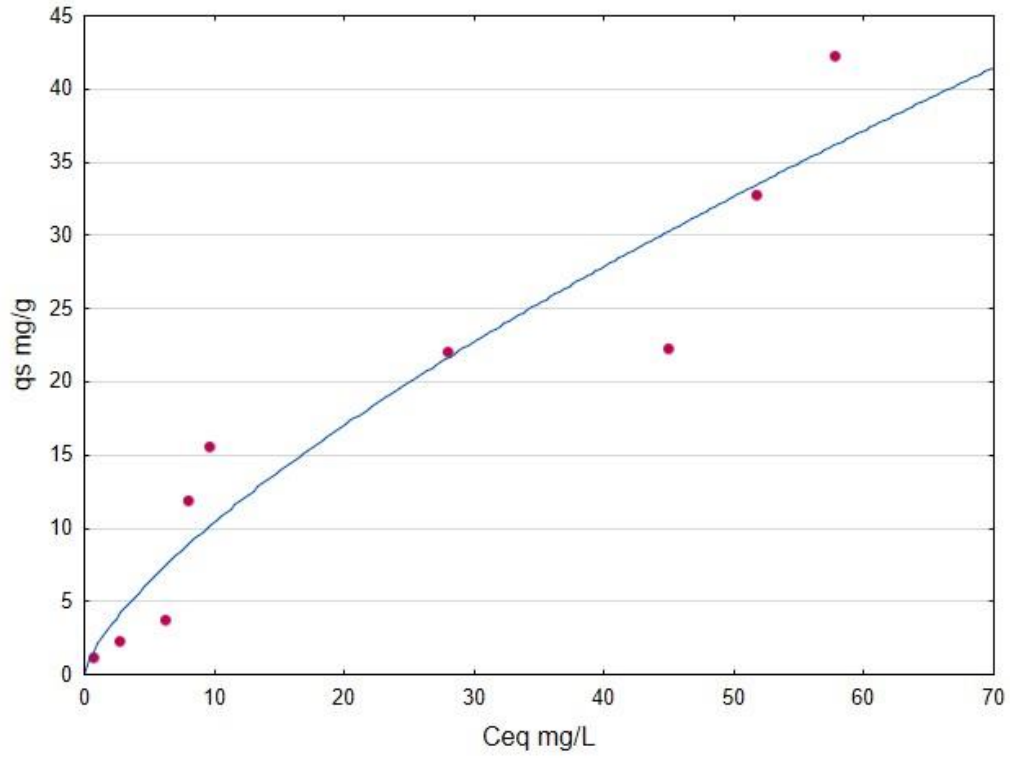
Fig. A6 DCF - BCHSL Freundlich non-linear isotherm
