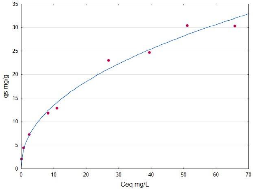
Fig. A12 MTP - BCHTH Freundlich non-linear isotherm
