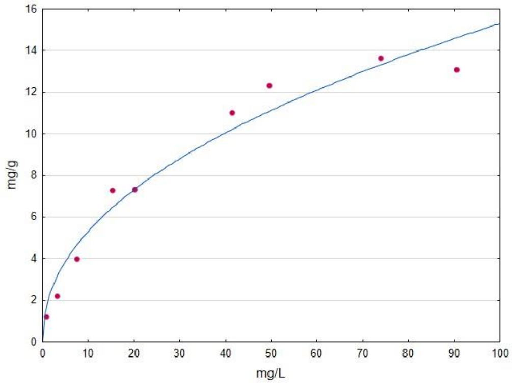
Fig. A18 BTR - BCHTL Freundlich non-linear isotherm
