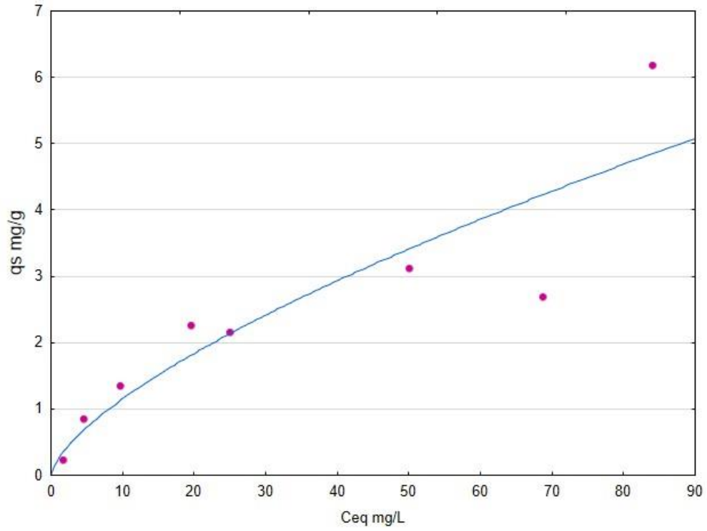
Fig. A2 DCF - BCHTL Freundlich non-linear isotherm
