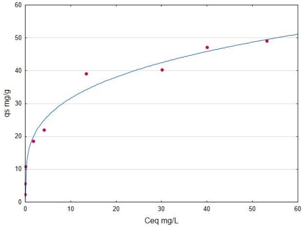
Fig. A8 DCF - BCHTL Freundlich non-linear isotherm
