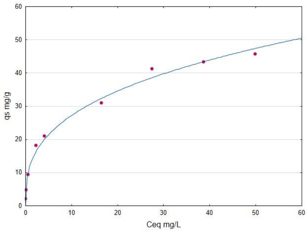
Fig. A14 MTP - BCHSL Freundlich non-linear isotherm
