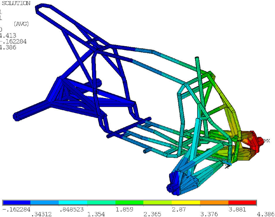
Obr. 32 Deformace modelu
