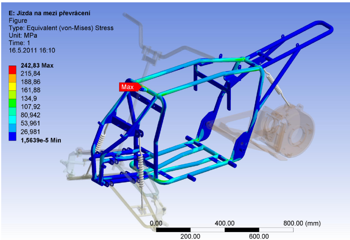
Obr. 38 Redukované napětí (von-Mises) při jízdním stavu průjezdu zatáčkou na mezi převrácení
