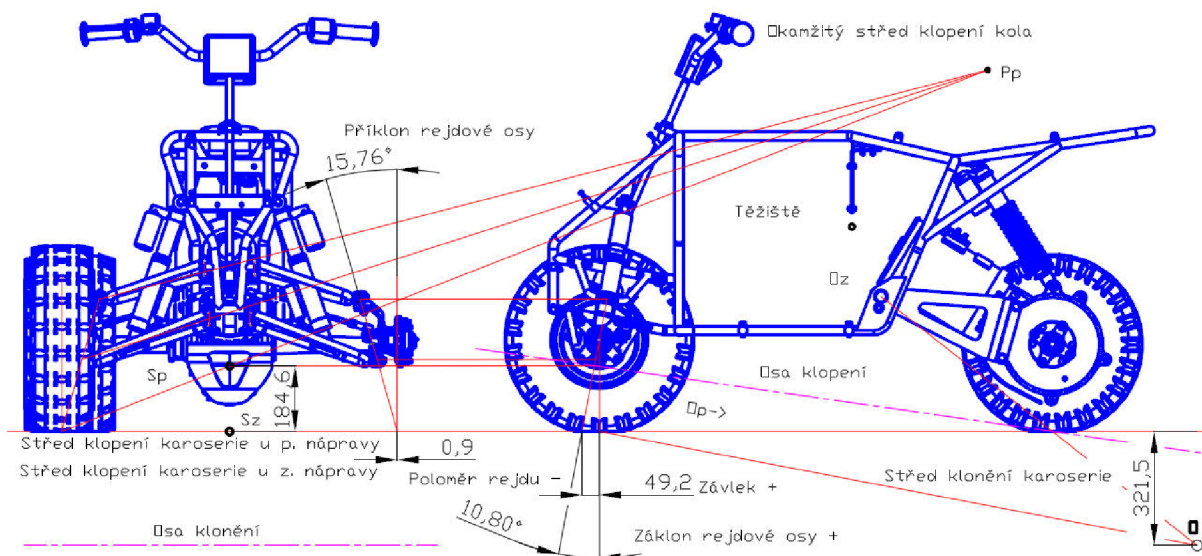
Obr. 46 Úhly zavěšení, středy klopení a klonění karoserie
