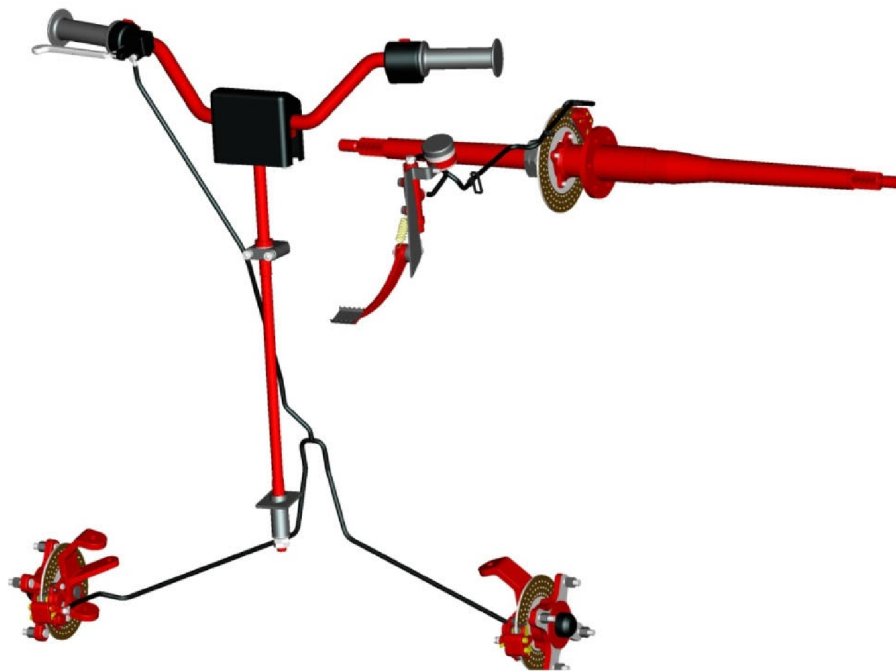
Obr. 77 Přední a zadní brzdový okruh
