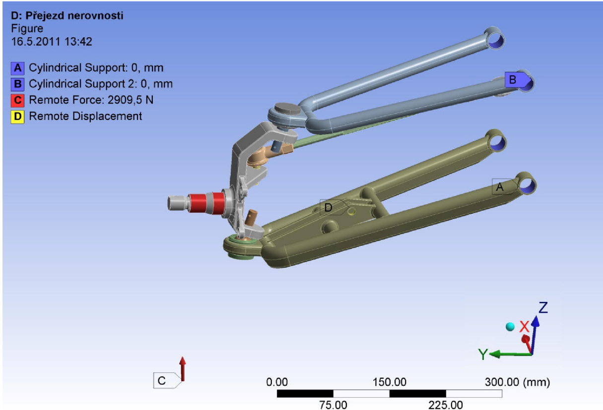
Obr. 56 Zatížení a zajištění nápravy proti pohybu pro stav přejezdu nerovnosti
