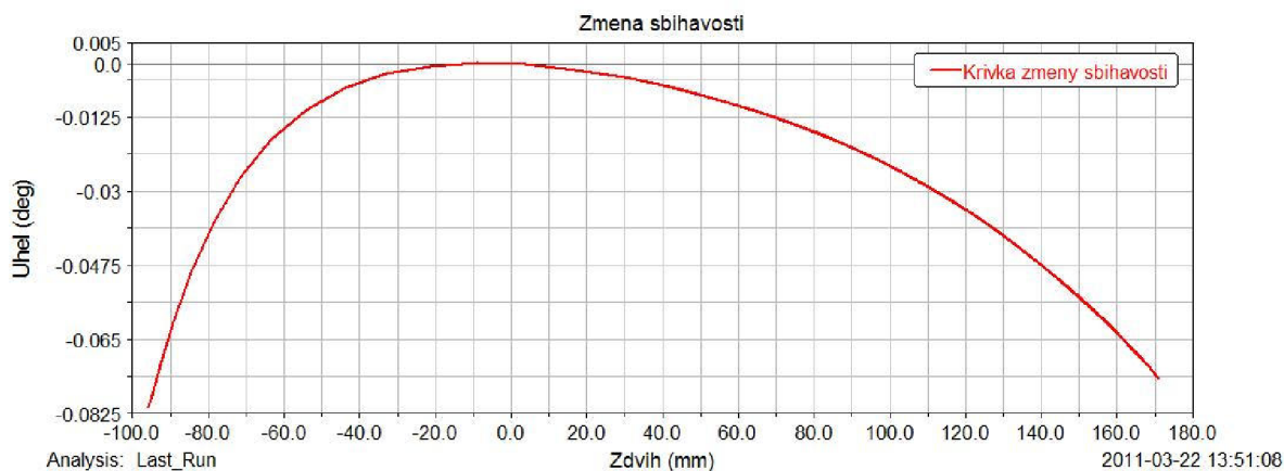
Obr. 42 Změna sbíhavosti
