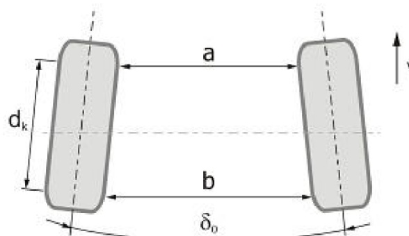
Obr. 41 Sbíhavost kol[18]
