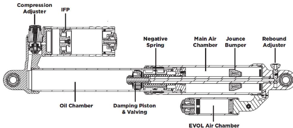
Obr. 54 Tlumič pérování Float X Evol [22]
