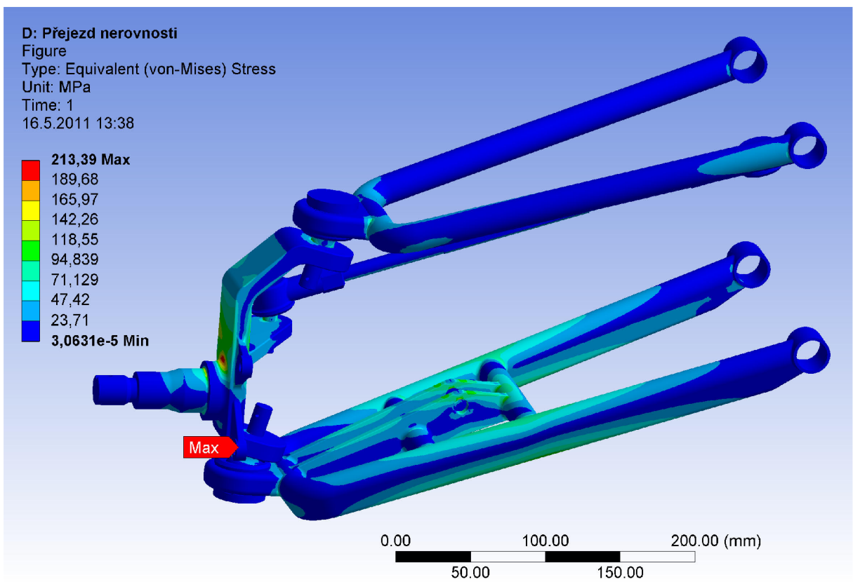
Obr. 57 Napětí na nápravě při přejezdu nerovnosti
