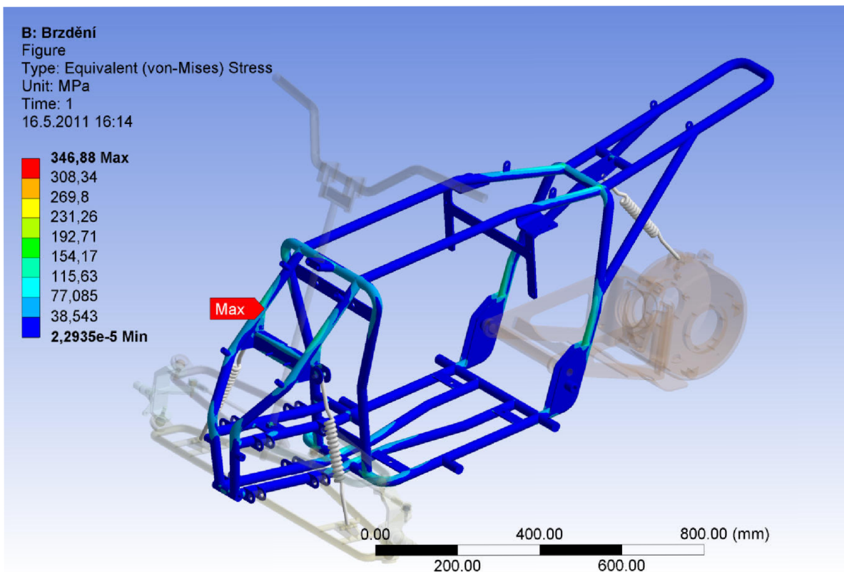
Obr. 34 Redukované napětí (von-Mises) pro jízdní stav brzdění
