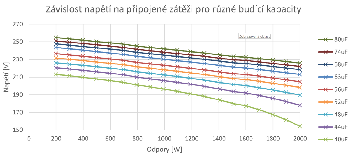
Obr. 4.1: Závislost napětí na zatížení při zvolené kapacitě
