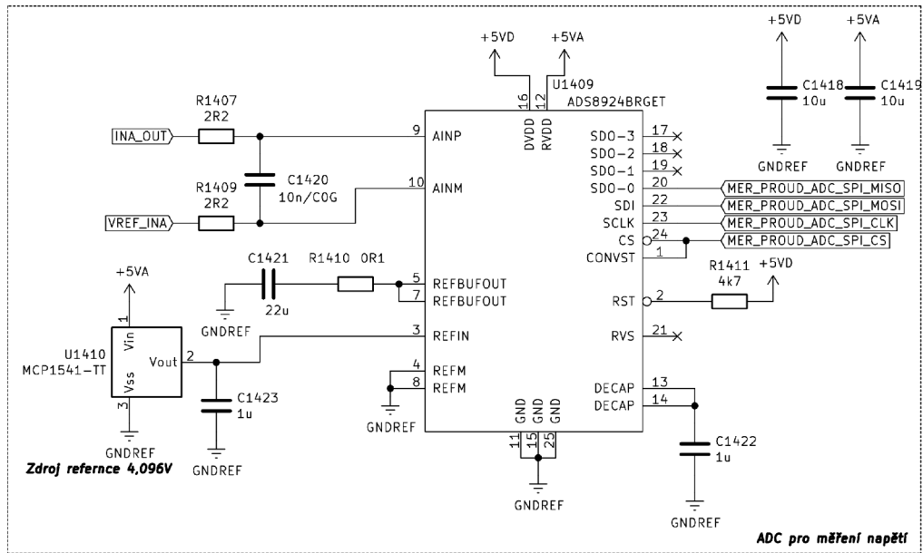
Obr. 8.16: Zapojení ADC pro měření výstupu z INA225
