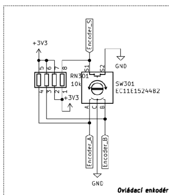
Obr. 8.24: Zapojení enkodéru s tlačítkem
