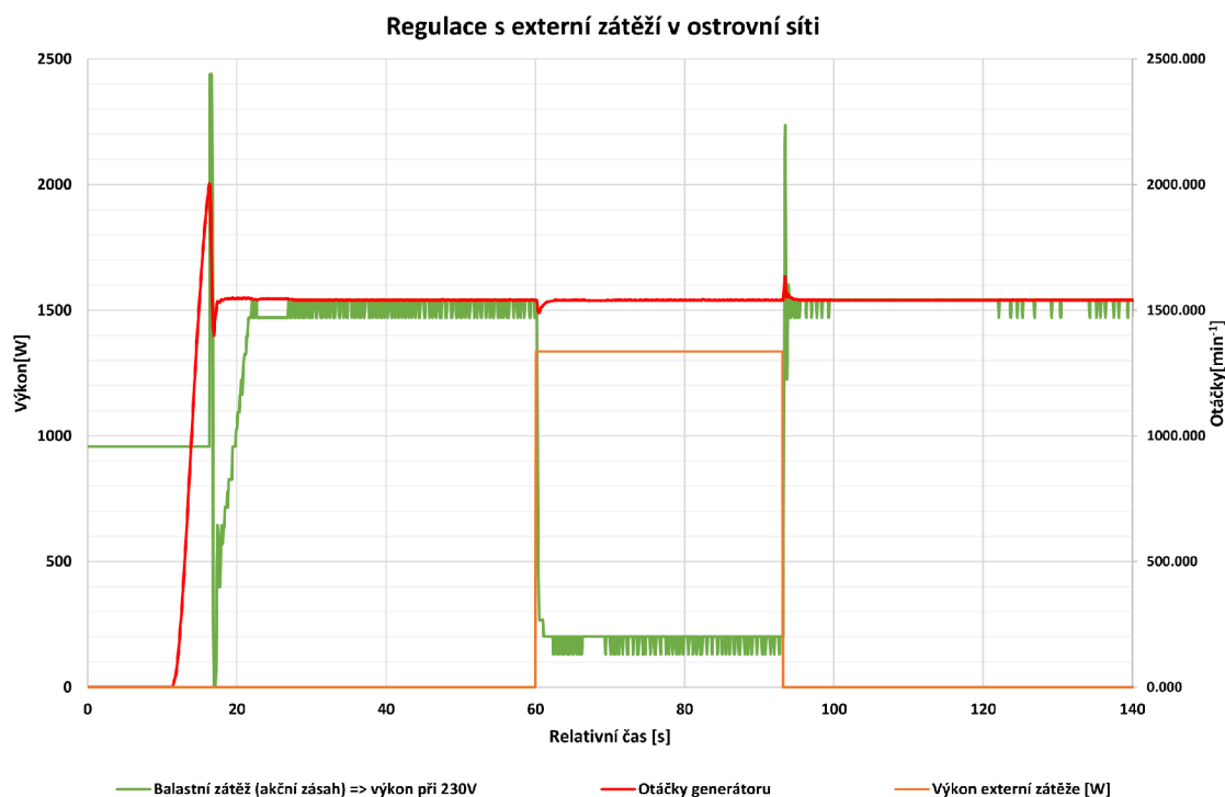
Obr. 11.5: Měřený průběh regulovaných otáček při zatěžování se změnou parametrů PSD regulátoru
