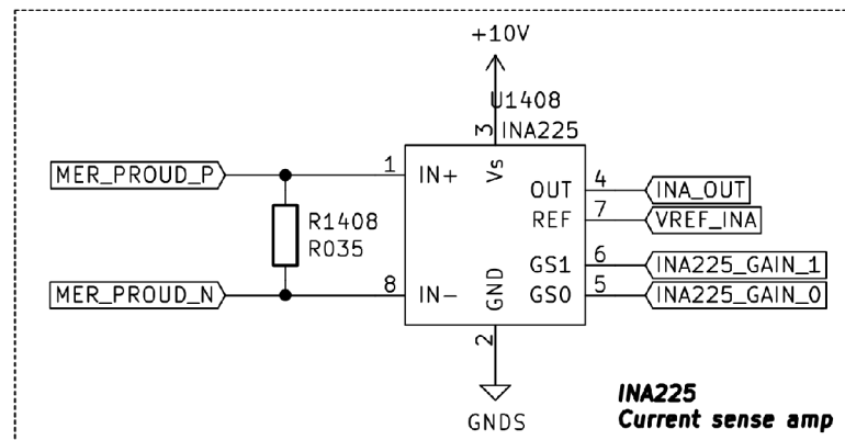
Obr. 8.13: Zapojení INA225
