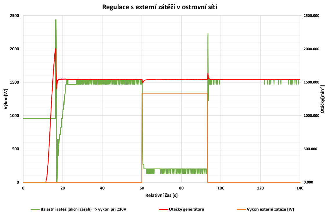
Obr. 11.8: Měřený průběh regulovaných otáček při zatěžování se změnou parametrů PSD regulátoru s PLC
