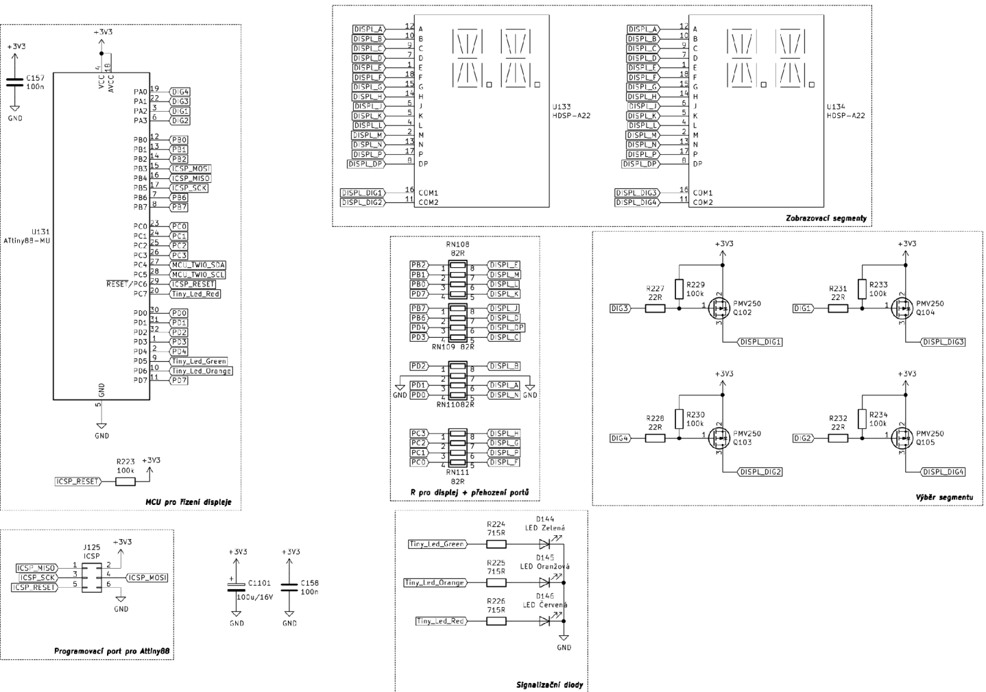
Obr. A.1: Zapojení displeje
