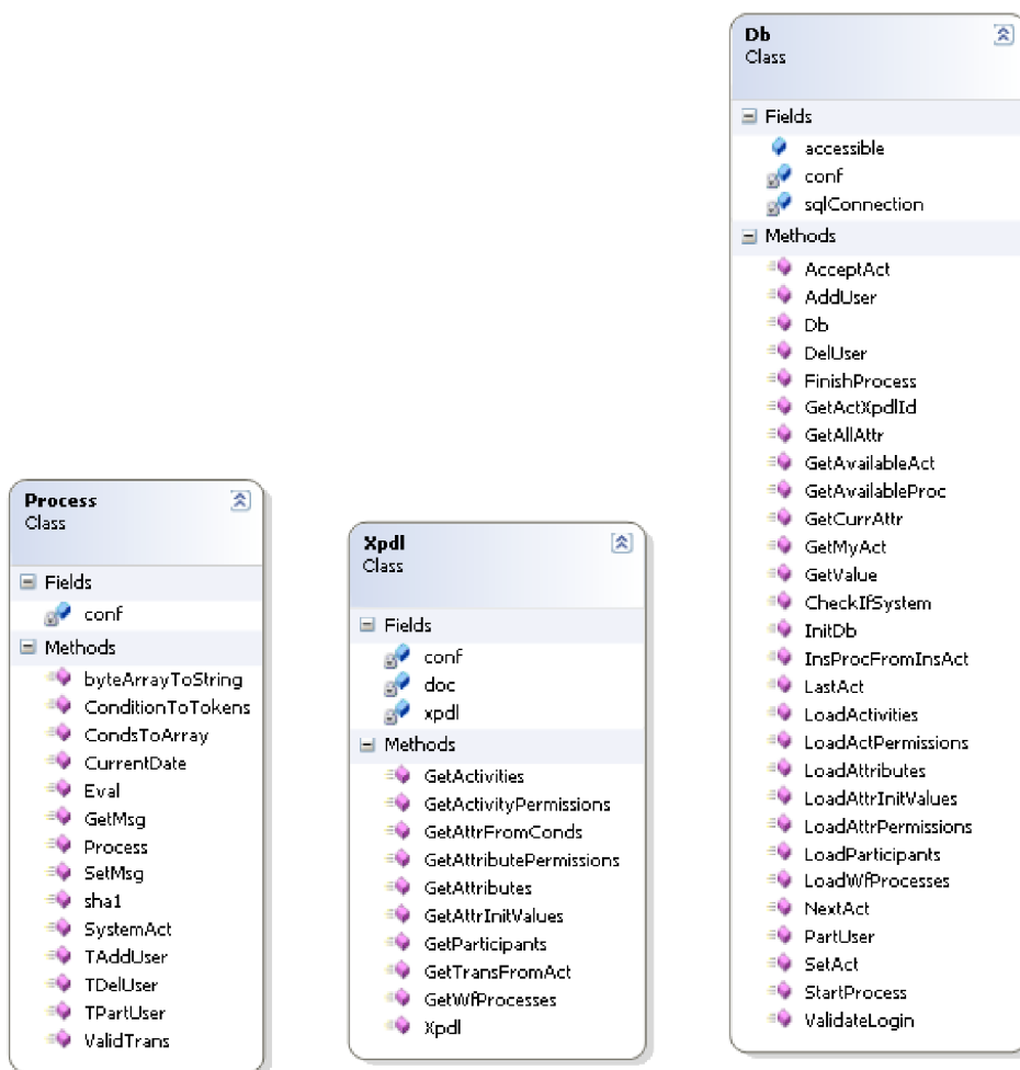
Obr. 8: Diagram tříd - jaderné třídy pro obsluhu databáze (Db), XPDL dokumentů (Xpdl) a vyřizování zpráv a dalších pomocných činností (Process)
