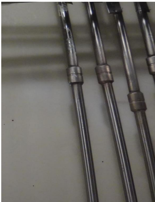
obr.2 Spoj s využitím převlečné trubky [2]
