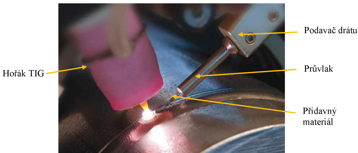
Obr. 8 Průběh svařování [8]
