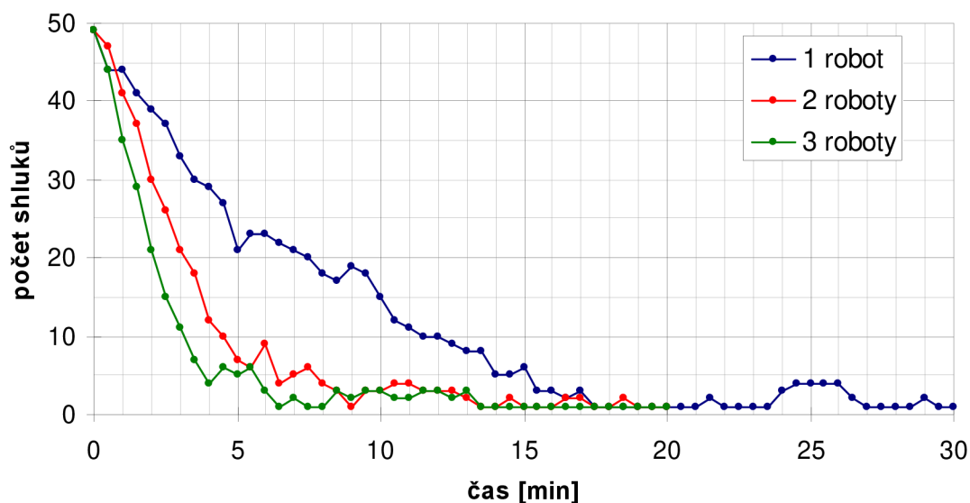
Obrázek 31 – Nejlepší časové průběhy počtu shluků
