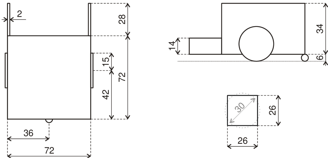
Obrázek 18 – Půdorys a nárys robotu a puku (rozměry v cm)
